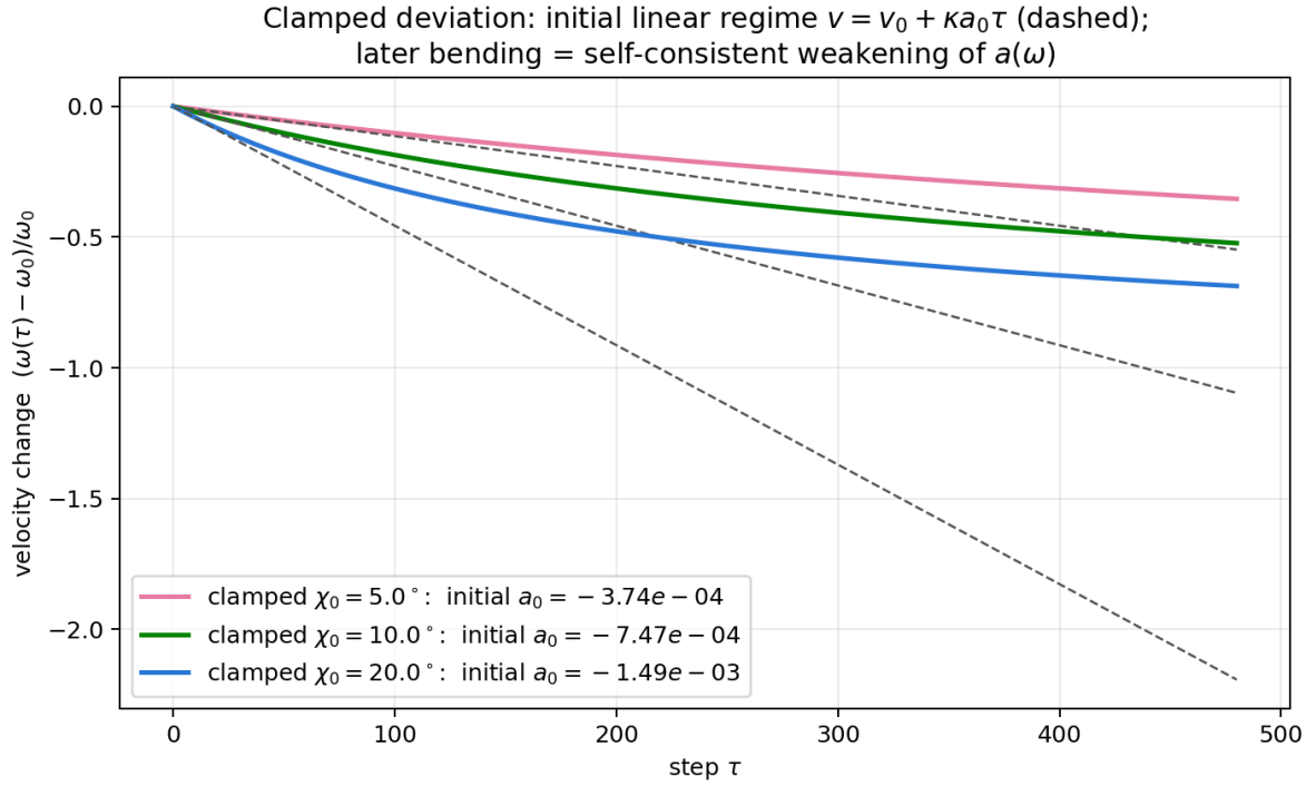
図 J2 は、偏差を拘束して a をほぼ一定にした対照である。キャリア速度は初期に v = v_0 + \kappa a_0 \tau の直線（破線）で成長し、後半の曲がり（実線）は速度変化が a(\omega) 自身を弱める自己無撞着効果である。
