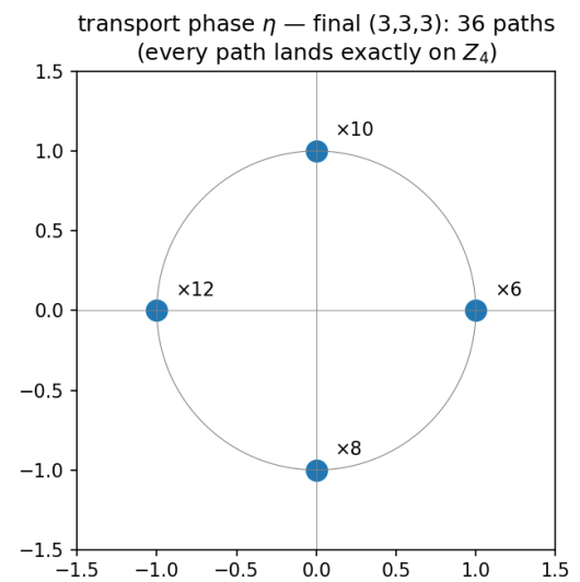
図2 輸送位相は例外なく Z_4 に着地
