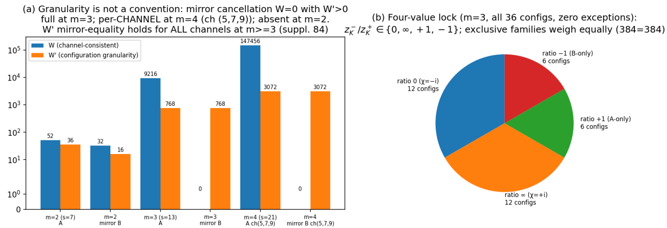
図4 干渉粒度の非規約性と四値ロック
