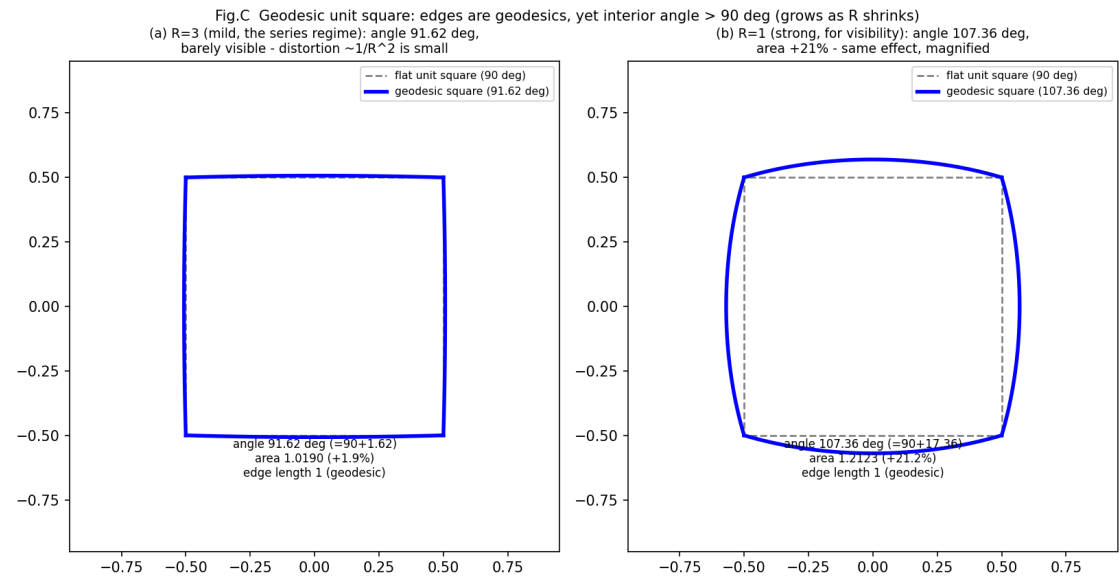
図 C. 測地正方形の角超過。辺長 1 の測地正方形 (各辺は測地線=その空間の直線) でありながら内角は 90^\circ を超える。左: R=3 (シリーズの領域、 91.62^\circ ではほぼ平坦、歪み \propto 1/R^2 は小さい)、右: R=1 (視認用、 107.36^\circ ・面積 +21%、同じ効果が拡大)。歪みは辺長でなく角と面積に現れ、 R が小さいほど大きい。
