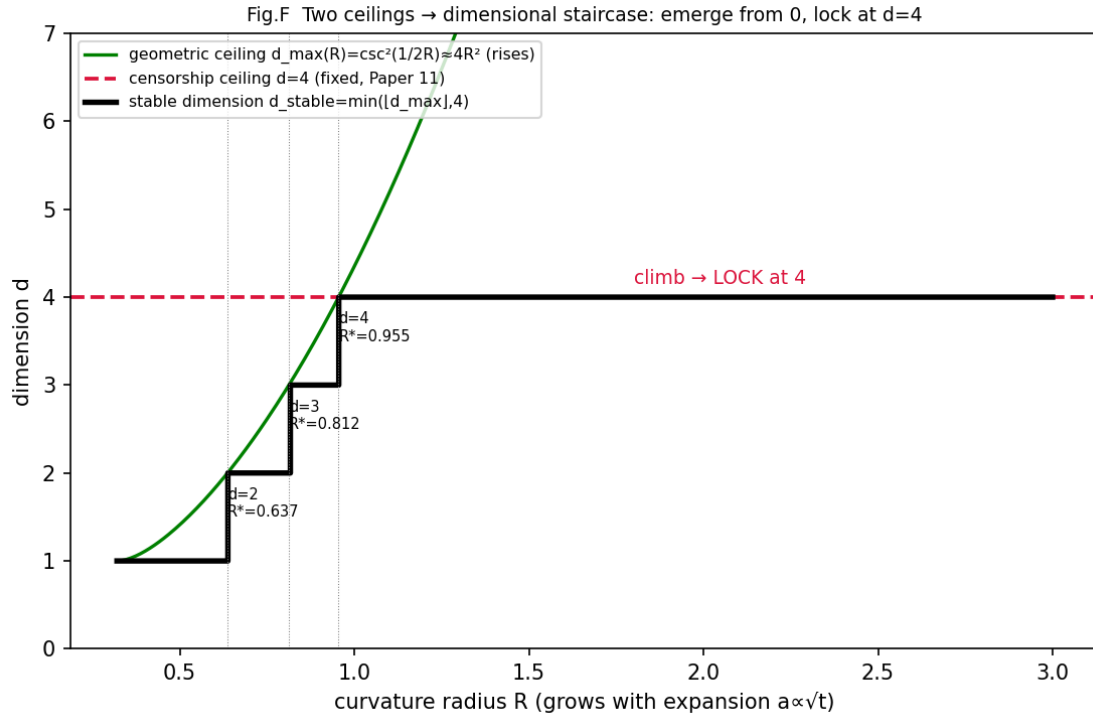
図 F. 次元の階段 (§4.7)。上昇する幾何天井 d_{\max}(R) \approx 4R^2 (緑) と固定の検閲天井 d=4 (赤破線、論文 11) の小さい方が安定次元 (太線)。R の増大 (膨張) とともに 1 \rightarrow 2 \rightarrow 3 \rightarrow 4 と登り、 R \geq 3/\pi で 4 にロックする。
