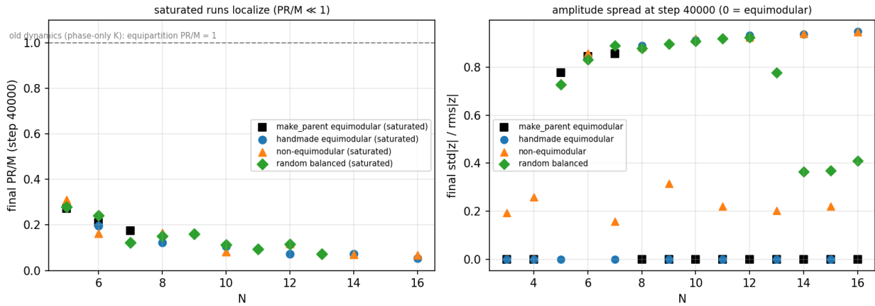
図 8. step 40000 の状態。左：飽和した走行の参加率 PR/M—破線の PR/M = 1 (旧力学の等分配) に達するものではなく、 N とともに 0.3 から 0.05 へ下がる。右：振幅の広がり \text{std}|z|/\text{rms}|z| —飽和した走行は生成法によらず 0.7 \sim 0.95 に集まり、床の走行は初期値 (等モジュラーなら 0) のまま。
