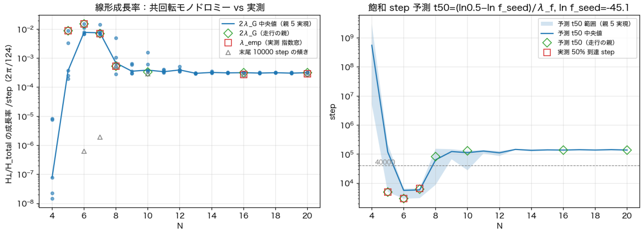
図 11. make_parent 等モジュラー親 (各 N 5 実現) の成長率と飽和 step。左：共回転 1 刻み線形化行列の 2\lambda_G (青、中央値と実現ごとの点) と実測 \lambda (赤四角) — N \geq 9 で 3 \times 10^{-4}/\text{step} の共通床 (刻み由来項) に張り付く。右：予測 t_{50} = (\ln 0.5 - \ln f_{\text{seed}})/\lambda_f と実測 — N = 5 \sim 7 は 40000 以下、 N \geq 8 は 10^5 以上。 \tau 単位では \tau_{50} = 355/\Delta \rightarrow \infty ( \Delta \rightarrow 0 ) なので、中立な親は連続極限では飽和しない。§7 の「床」は 40000 step 内の判定であり、刻み由来の成長は 10^5 step 台で O(1) に達しうる。
