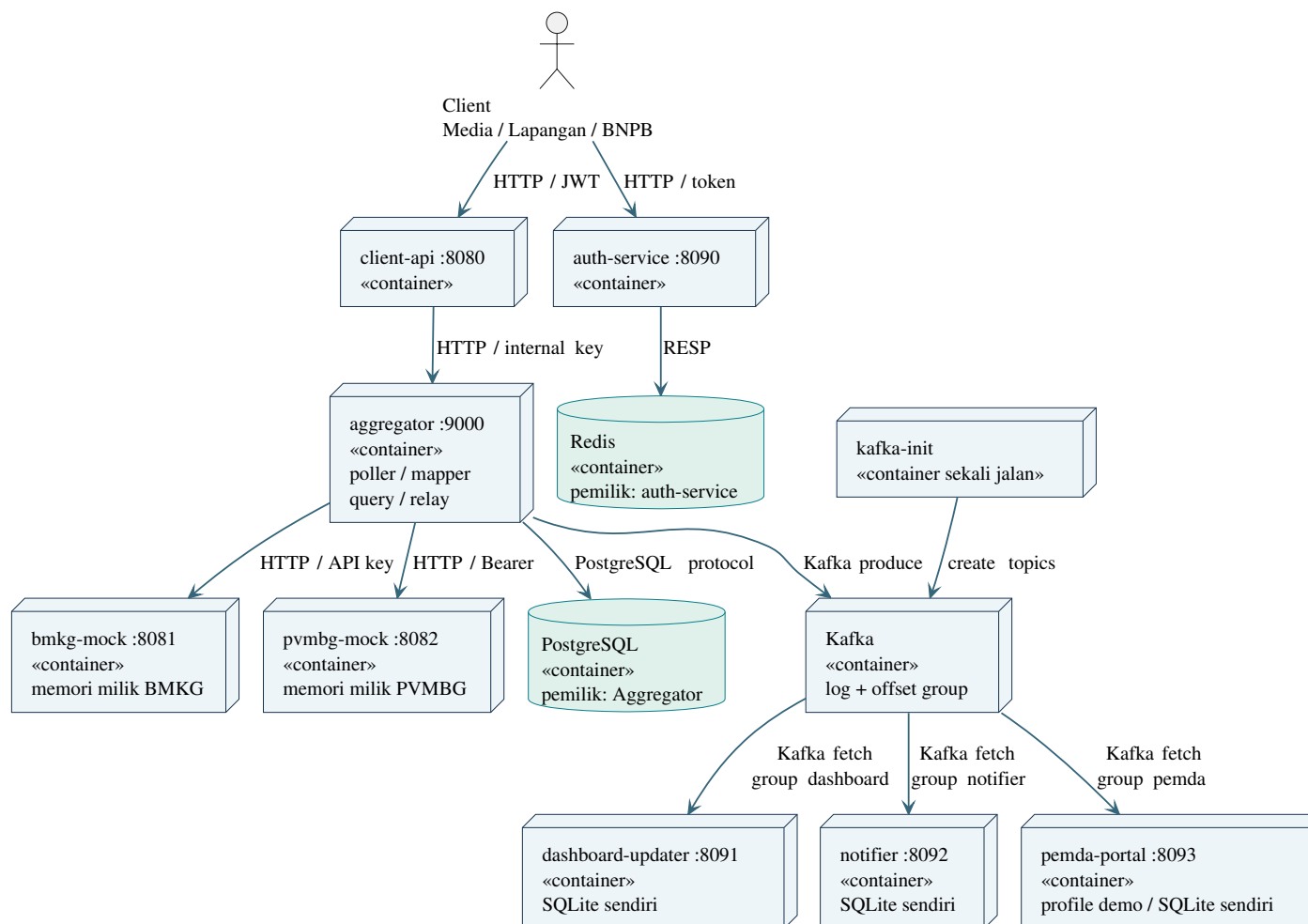
Gambar 1: Service, protokol, storage ownership, dan batas container. Memori mock dan SQLite berada pada container pemilik. Panah Kafka ke consumer menunjukkan aliran data; consumer menginisiasi fetch.
