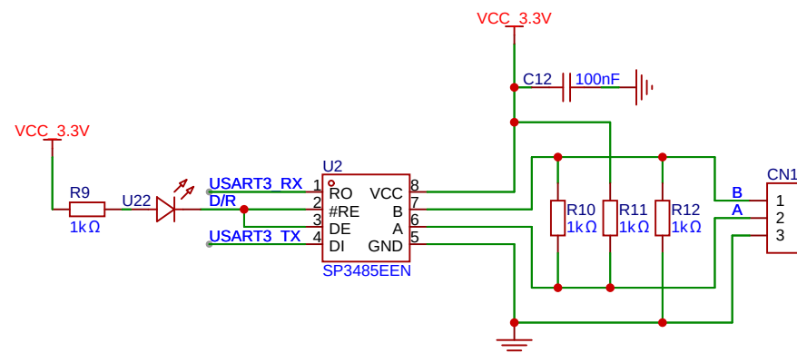
485通信
