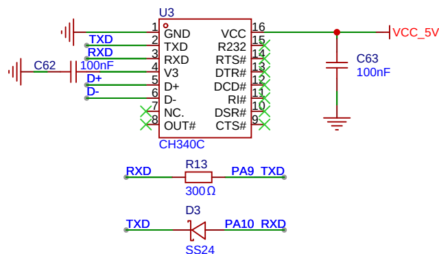
串口
