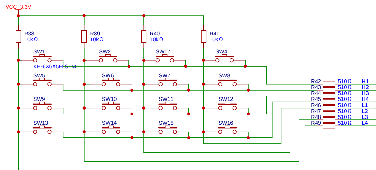
矩阵键盘
