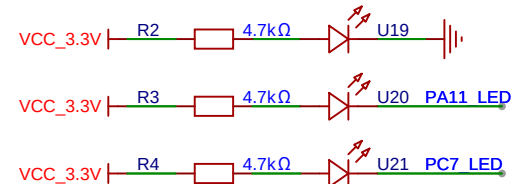
指示灯
