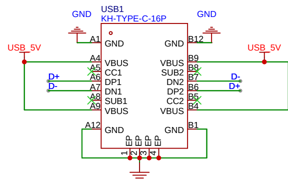
TYPE-C
