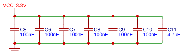
去耦电容
