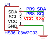
OLED屏
