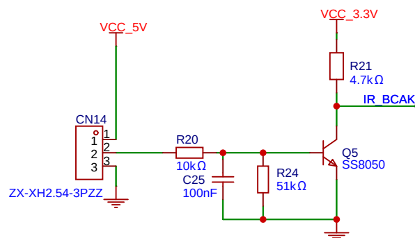
红外接收检测
