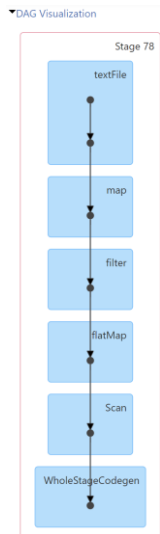
DAG
