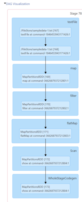
Optimisation DAG
