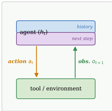
Coding-agent step
