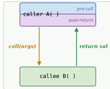
Function call site
