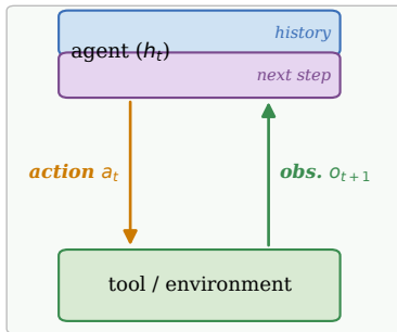
Coding-agent step
