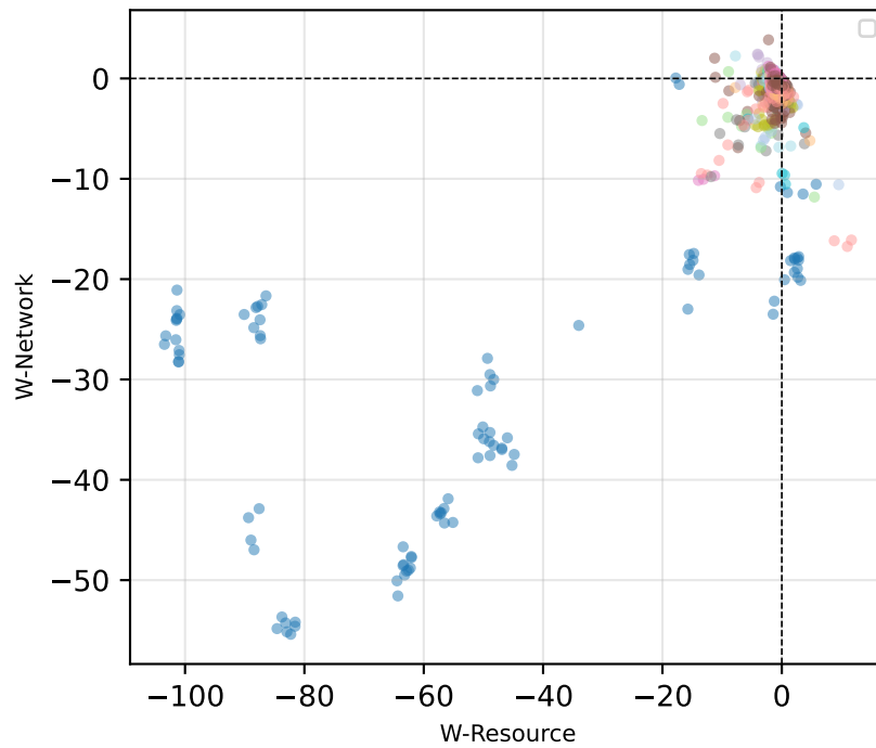
Regret (env ≠ ref)
