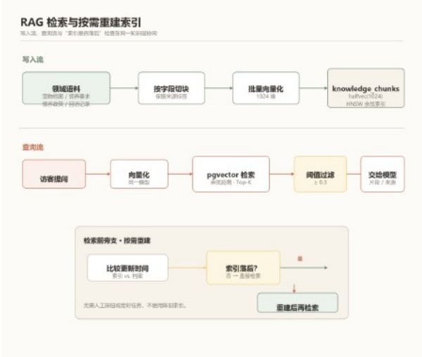
图 5 RAG 检索与按需重建索引
