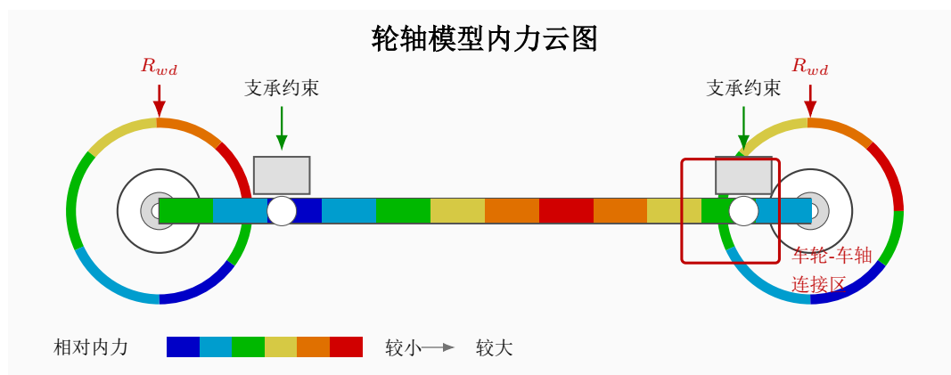
图 4-3 MIDAS 轮轴模型内力分布结果
