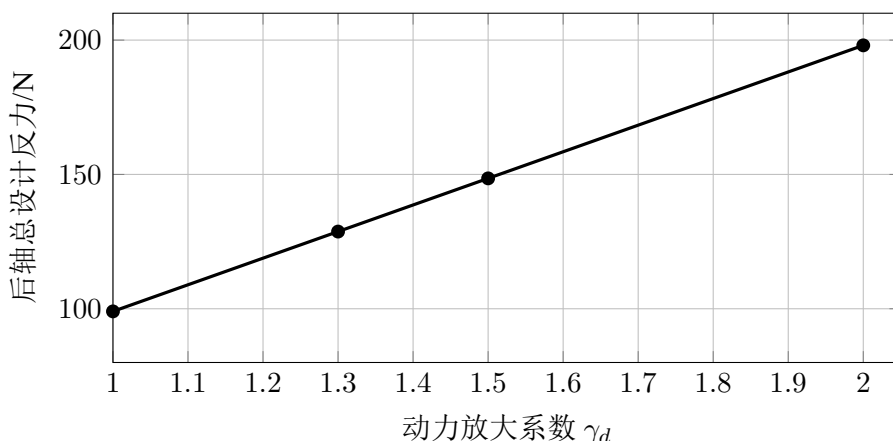
图 6-3 动力放大系数与后轴总反力关系
