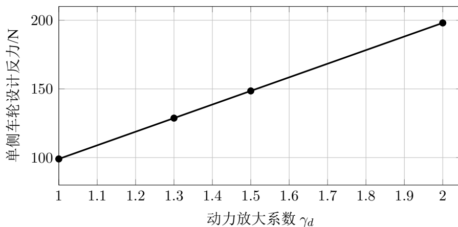
图 6-3 动力放大系数与车轮反力关系
