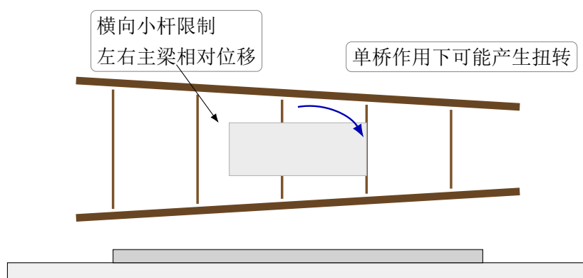
图 6-4 单桥工况下车架抗扭示意
