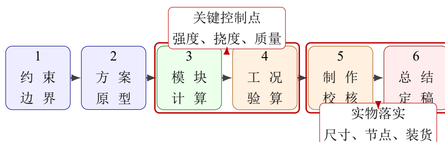
图 1-1 理论方案编制与实物校核流程
