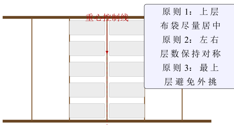
图 7-3 满载码放的重心控制示意
