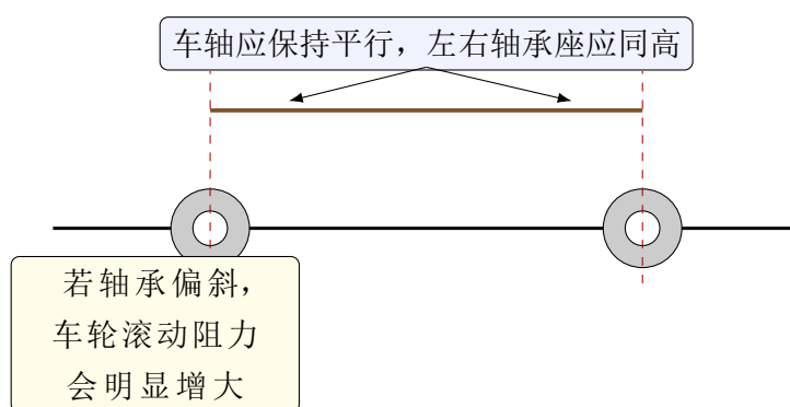
图 4-2 轮轴同轴度校正示意
