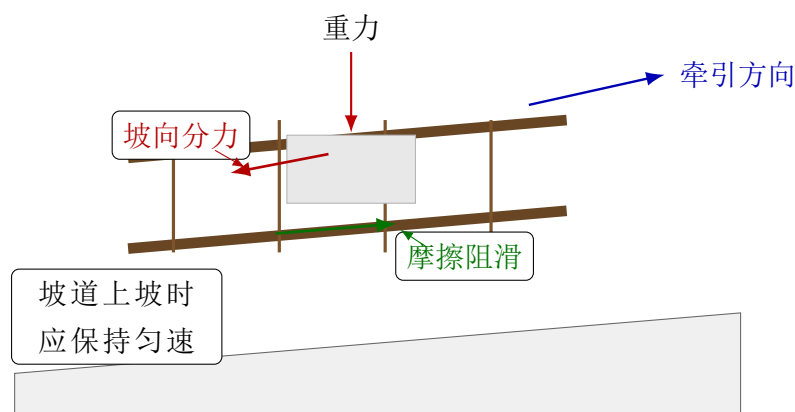
图 6-1 坡道牵引与布袋防滑示意
