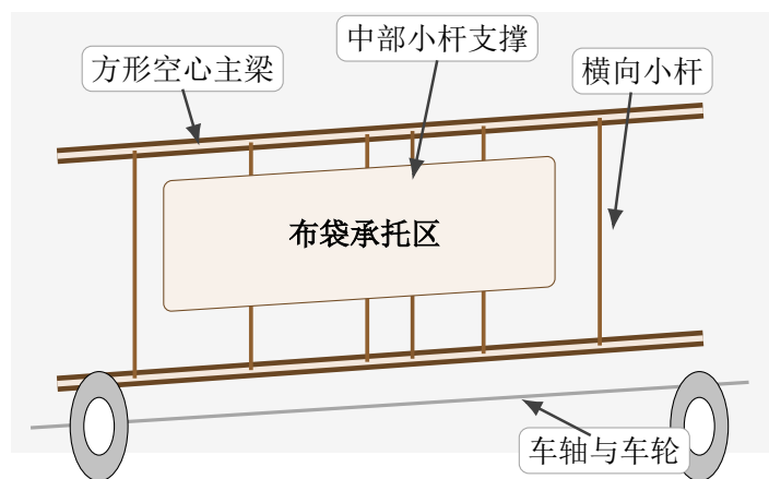
图 2-3 最终采用的空心双主梁勒勒车模型总体示意
