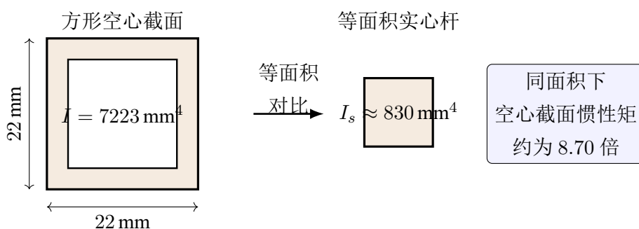
图 3-2 方形空心截面与等面积实心杆对比
