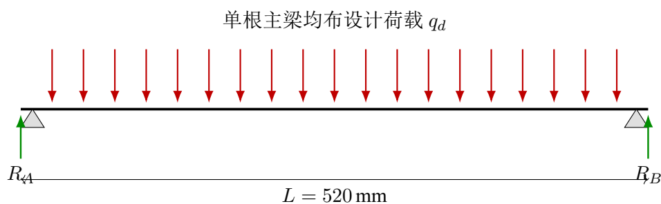
图 3-1 单根主梁等效简支梁模型
