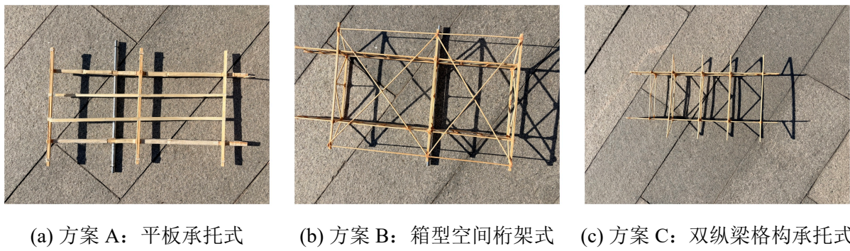
图 2-1 三种候选车架方案原型照片
