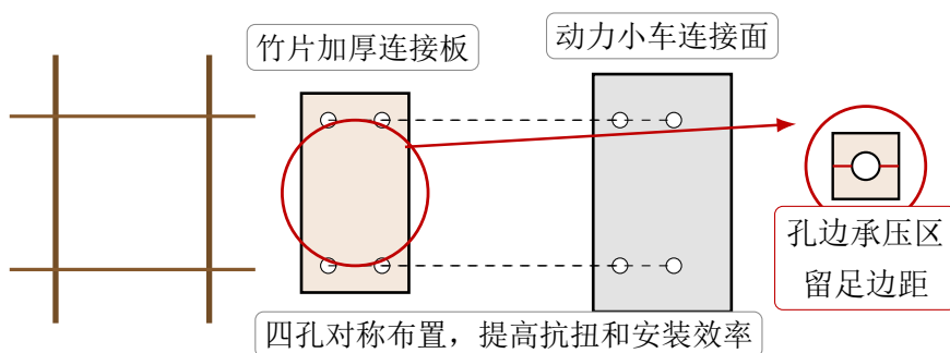
图 5-2 四螺丝牵引连接节点示意
