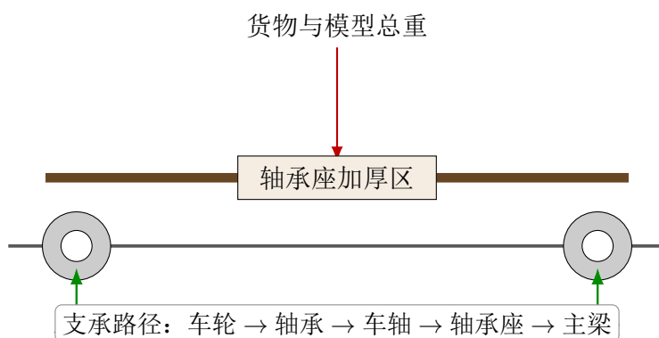
图 4-1 轮轴与车身支承反力示意
