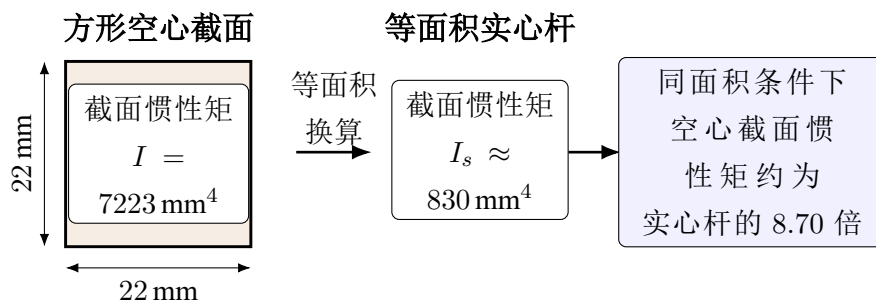
图 3-2 方形空心截面与等面积实心杆对比
