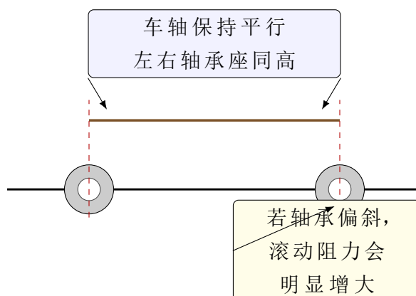
图 4-2 轮轴同轴度校正示意
