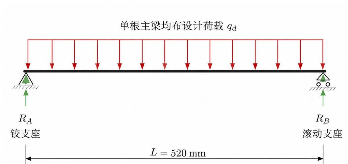
图 3-1 单根主梁等效简支梁模型
