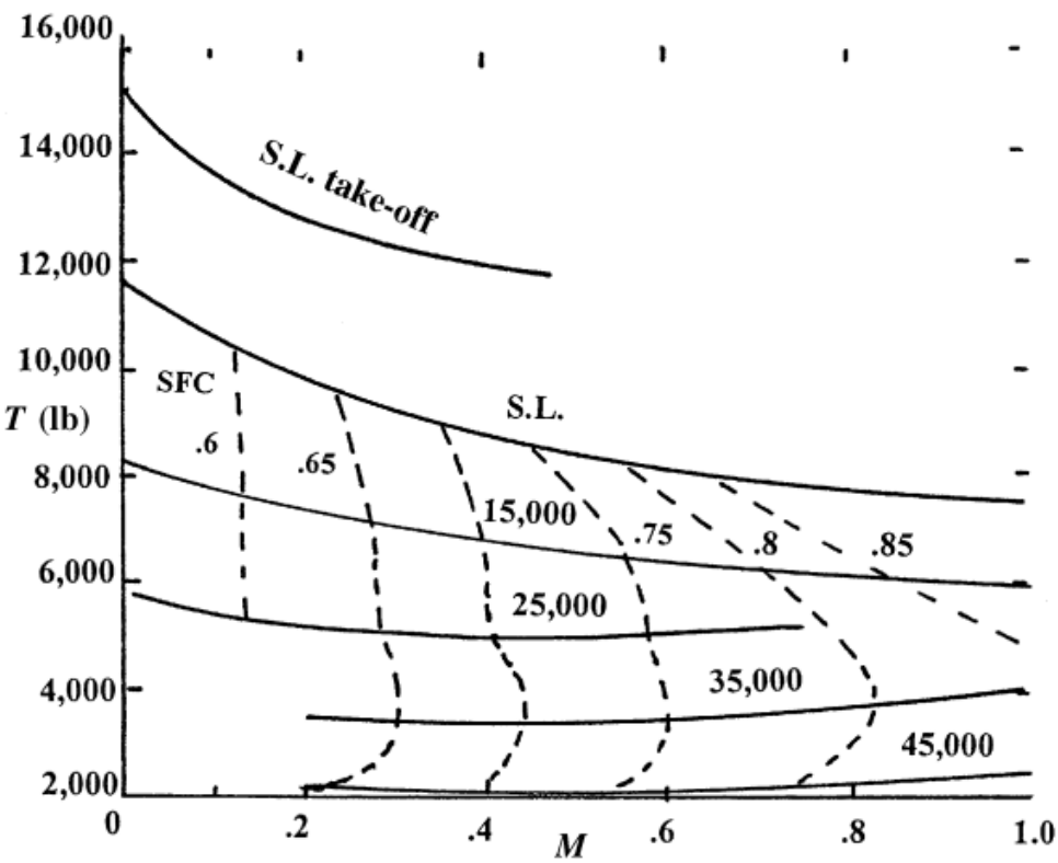
图1 普惠 JT8D-9 涡扇发动机推力及耗油率参数
