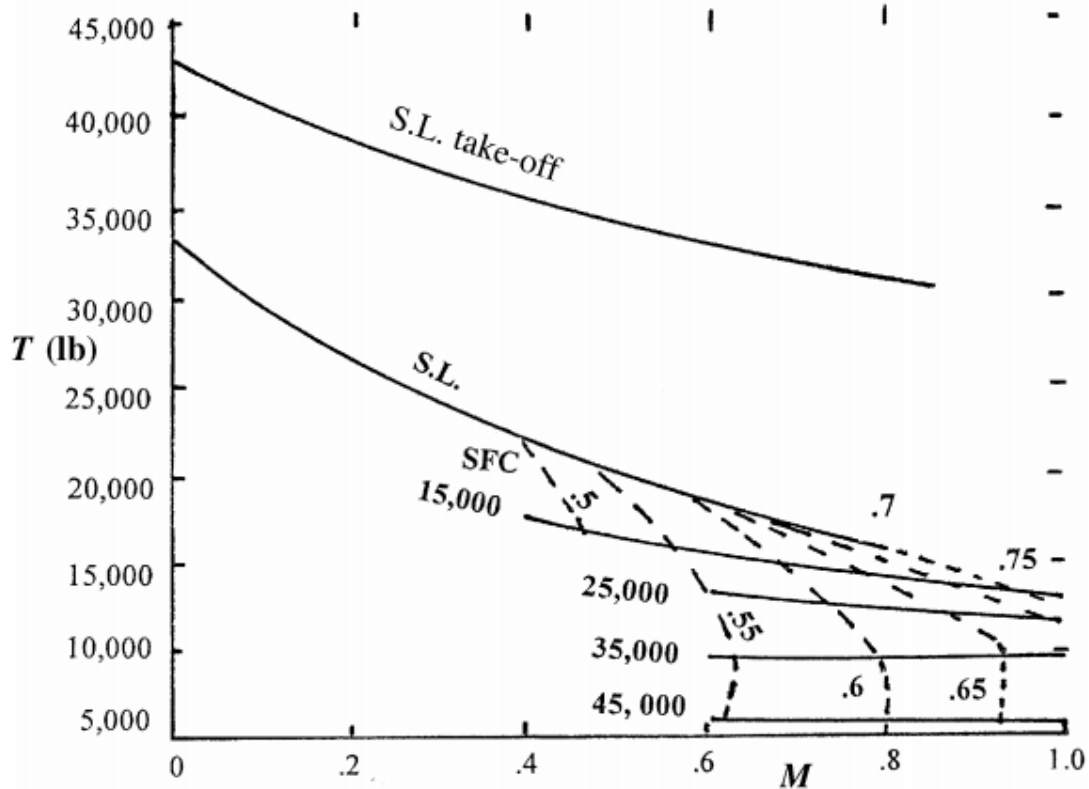
图2 普惠 JT9D-3 涡扇发动机推力及耗油率参数
