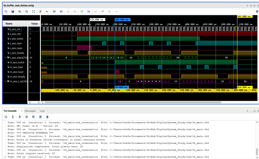
Figura 5.1: Waveform della simulazione: interazione tra FSM e Buffer Line durante la fase di Flush.
