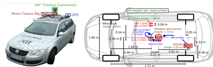
图 6: KITTI 数据采集平台。本报告中的所有实验都基于已归档的 KITTI Tracking 结果。
