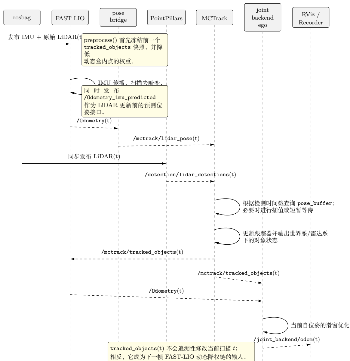
图 5: 在线优化链的执行级时序逻辑。当 FAST-LIO 处理当前 LiDAR 帧时, 它使用的是前一帧冻结下来的 tracked_objects 快照。MCTrack 在当前帧产生的跟踪结果, 主要会在下一帧进入动态降权链路。
