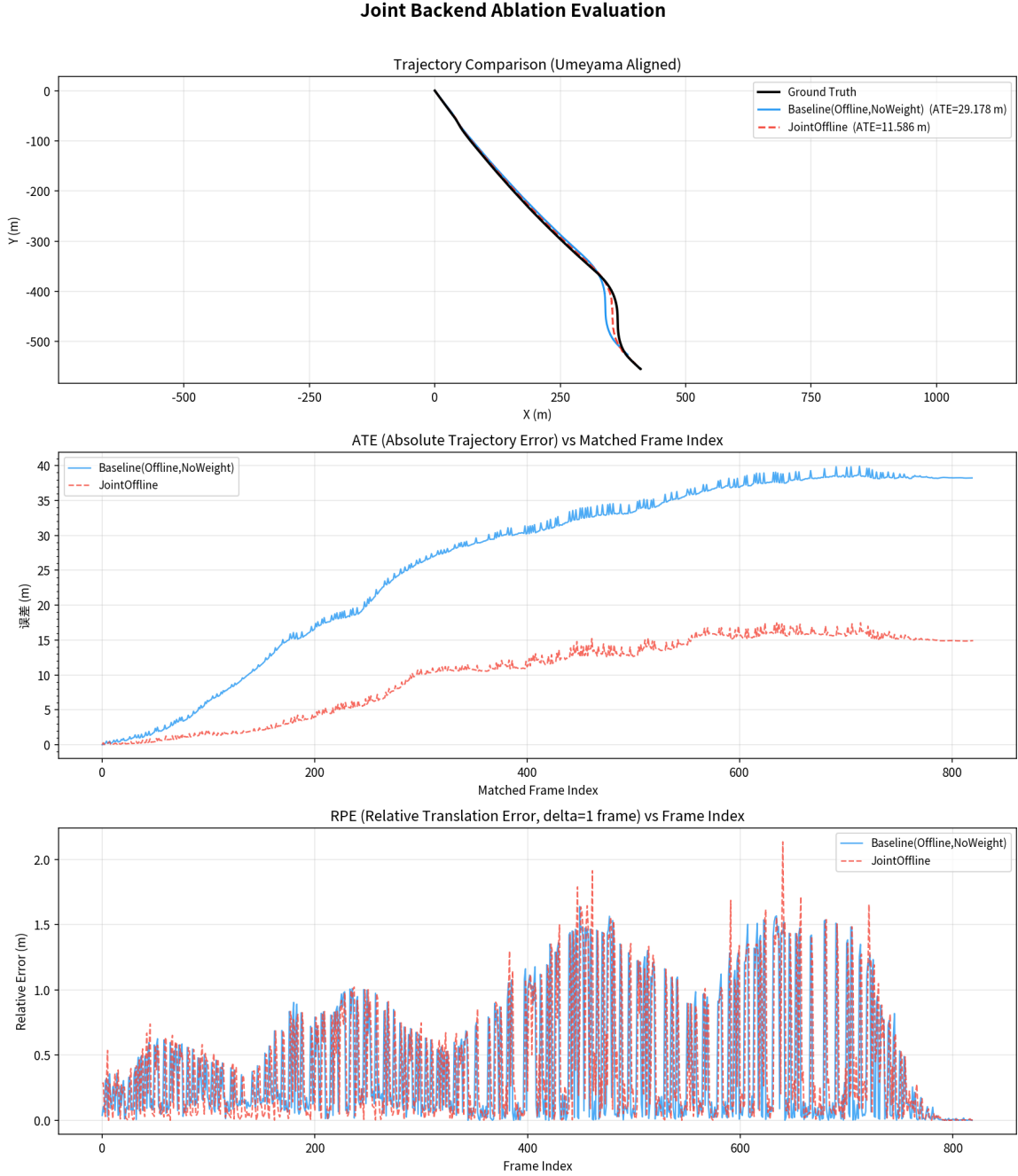
图 1: 序列 0020 的联合后端评估图。上图为 Umeyama 对齐后的轨迹对比，中图为 ATE 随帧变化，下图为单帧平移型 RPE。可以看到完整系统显著降低了全局漂移，但对局部 RPE 的改善不如 ATE 那样统一。
