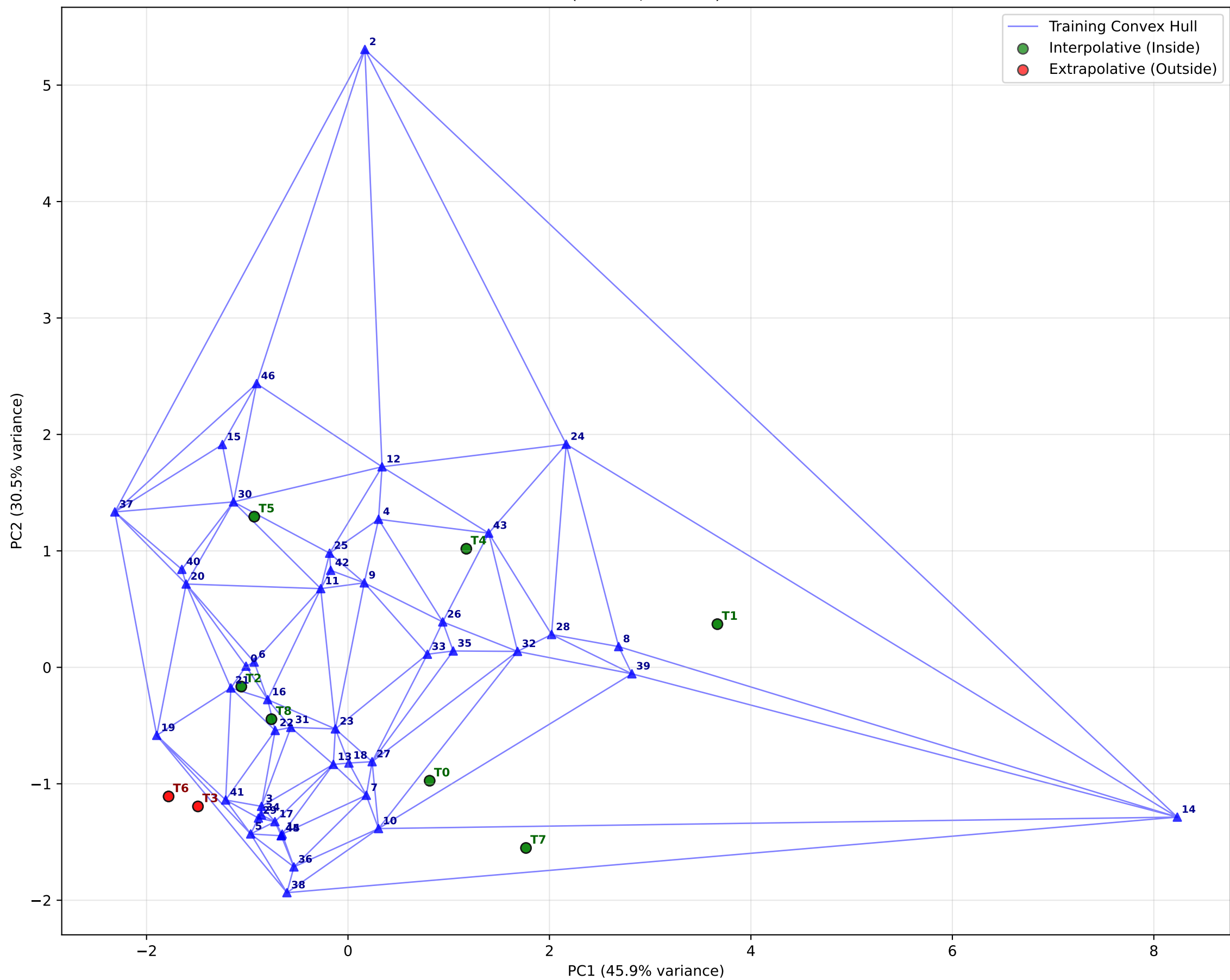
: Delaunay Triang (Train #, Test T#)
