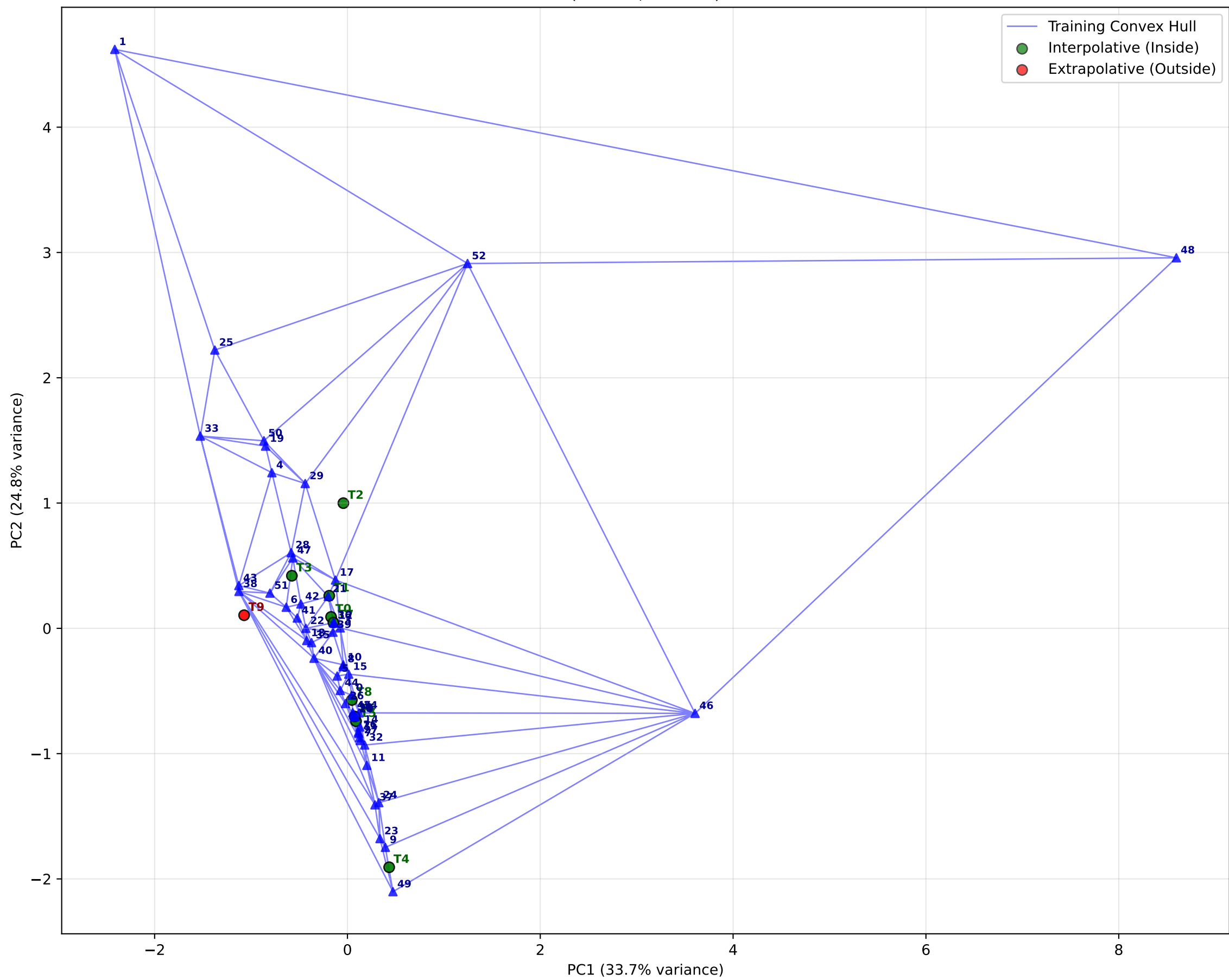
(Train #, Test #)
