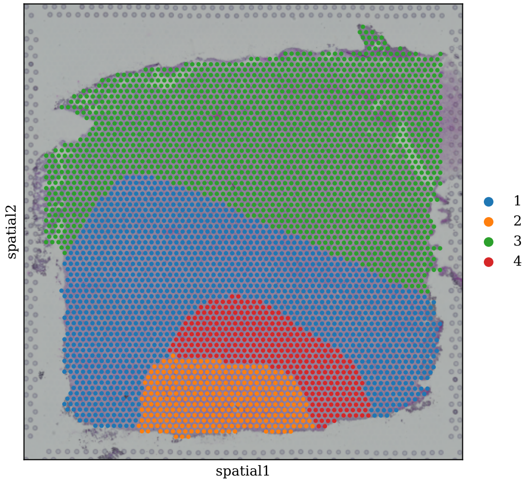
INR+PCA (Slice 151671)
