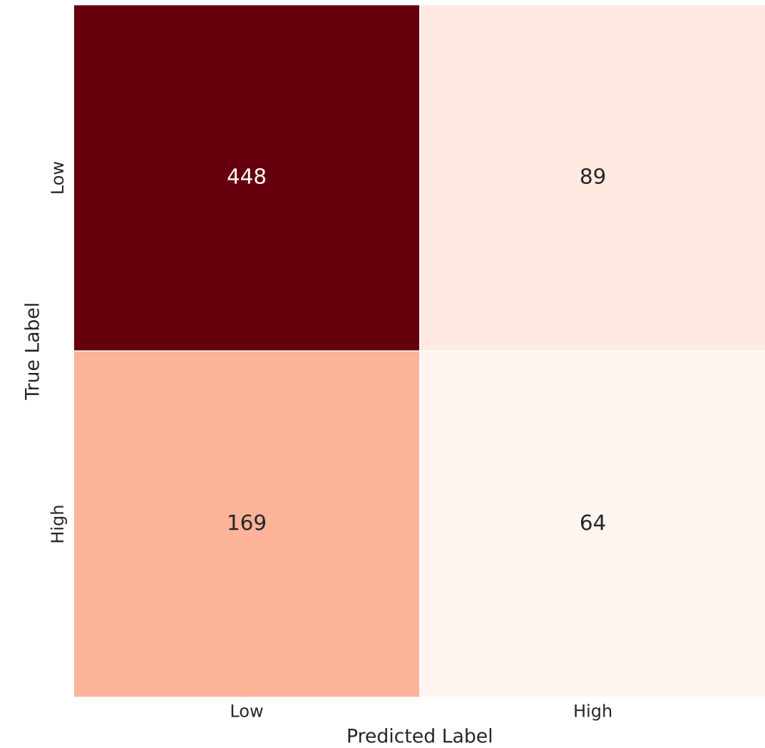
XGBoost (Fusion)
