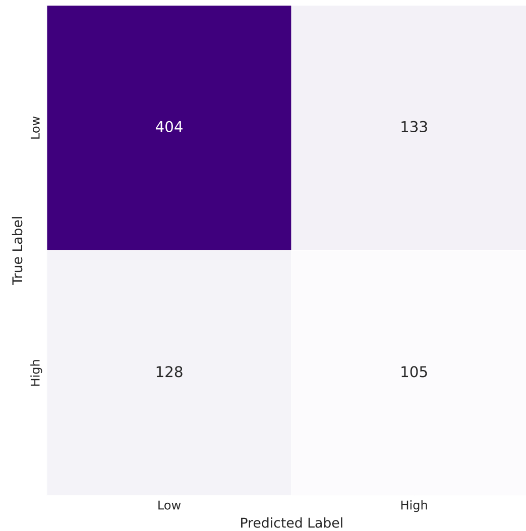
LR (Fusion)
