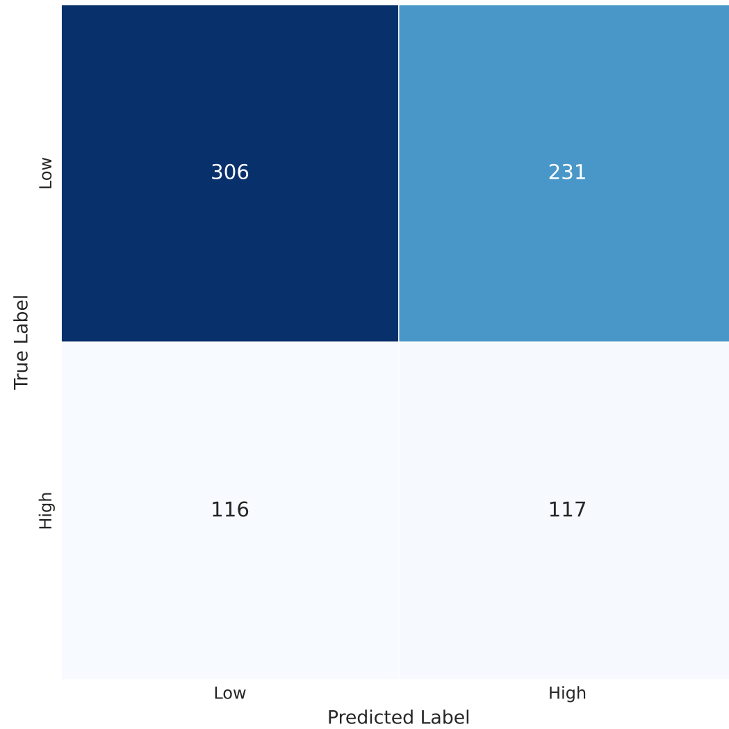
LR (WSV)
