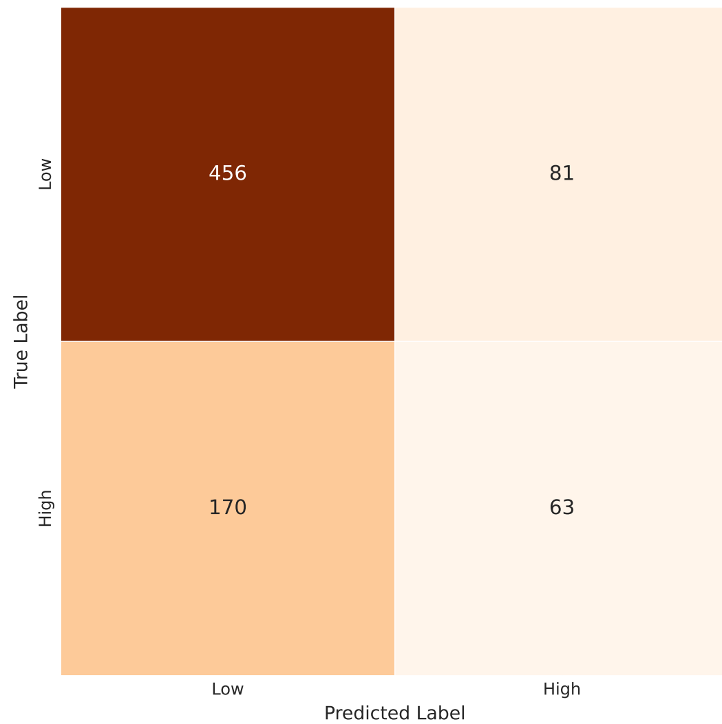
LR (WSV)
