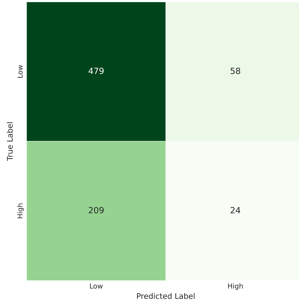
LR (Fusion)
