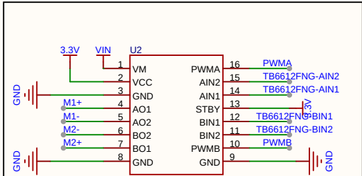
TB6612FNG电机驱动模块
