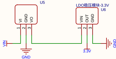
转3.3V
