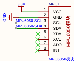
MPU6050
