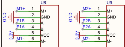
电机编码器
