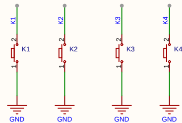
四个开关
