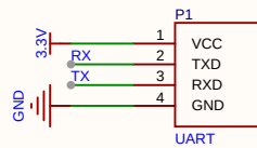
UART接口
