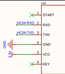
HC-04蓝牙
