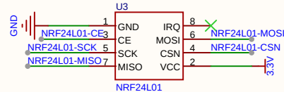
NRF24L01无线通讯模块
