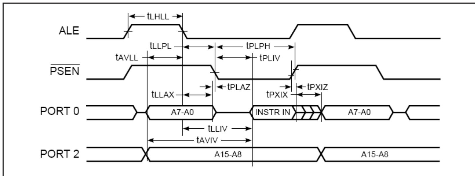
AT89C52的对外访问时序—程序存储器访问
