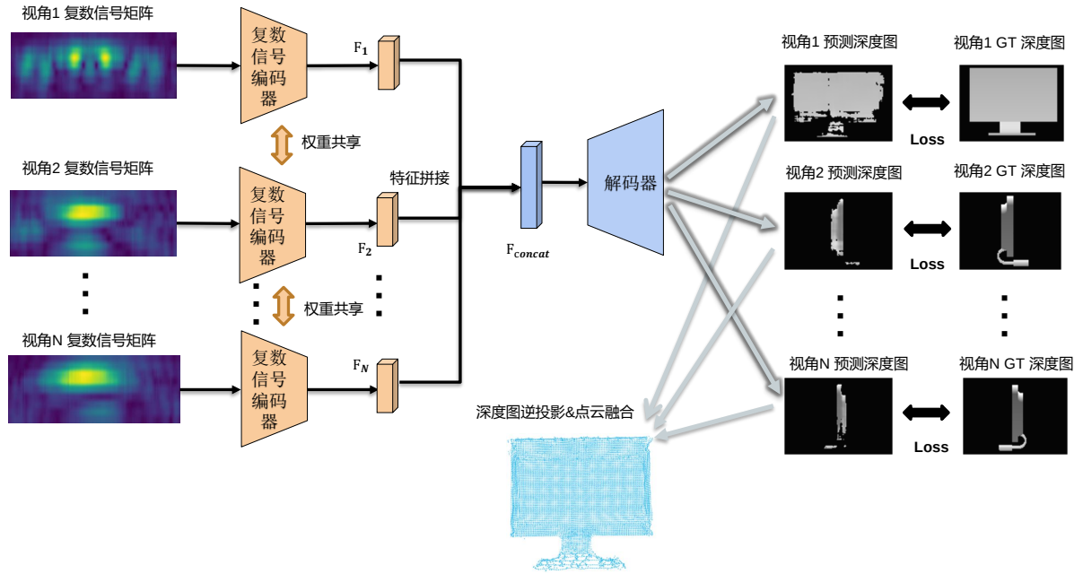
图 3-9 三维重建神经网络模型
