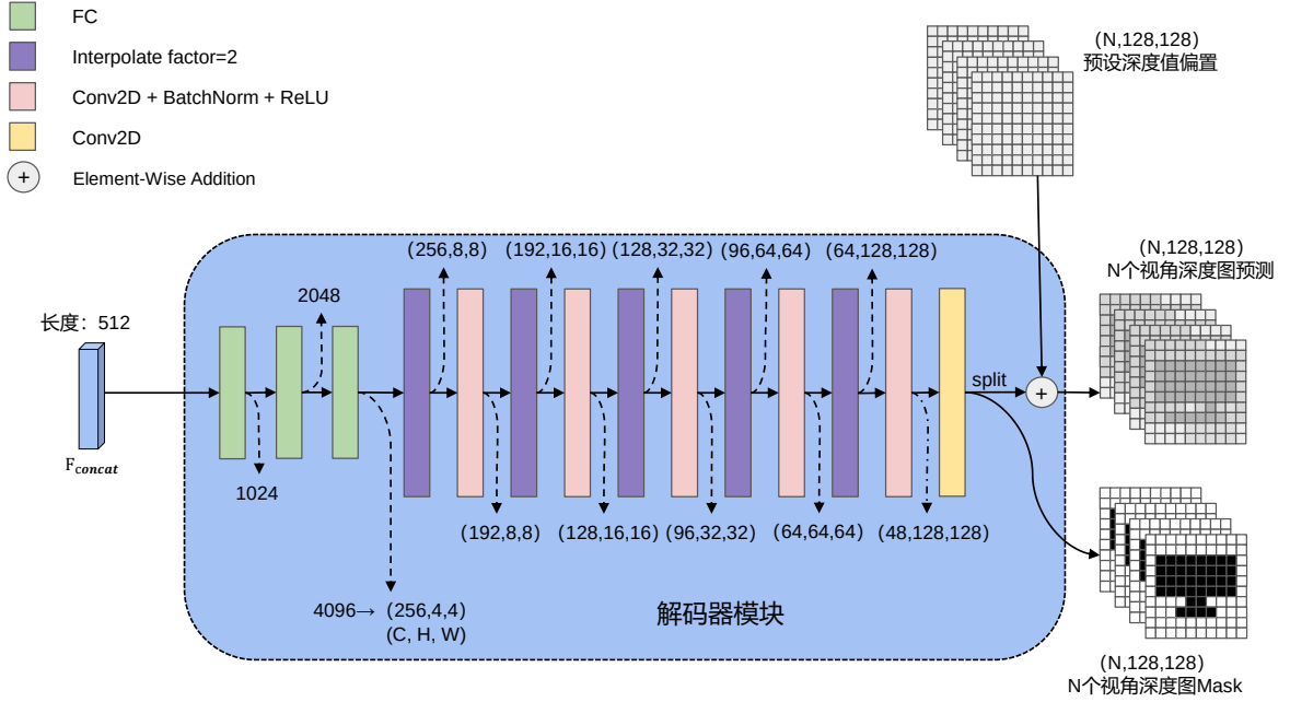
图 3-12 解码器模块
