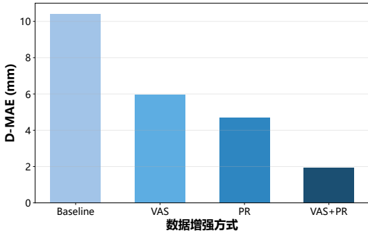
(a) D-MAE 对比 (越小越好)
