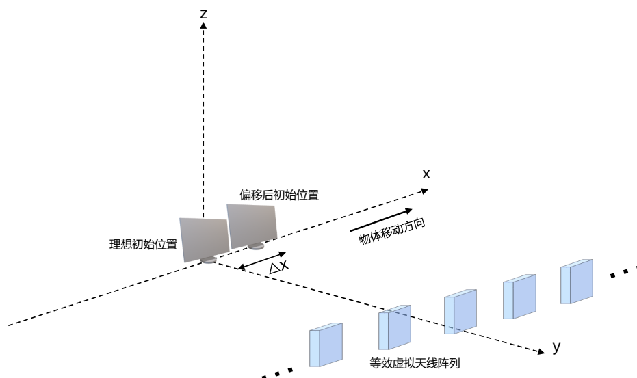
图 3-5 物体初始位置沿物体运动方向发生微小位移
