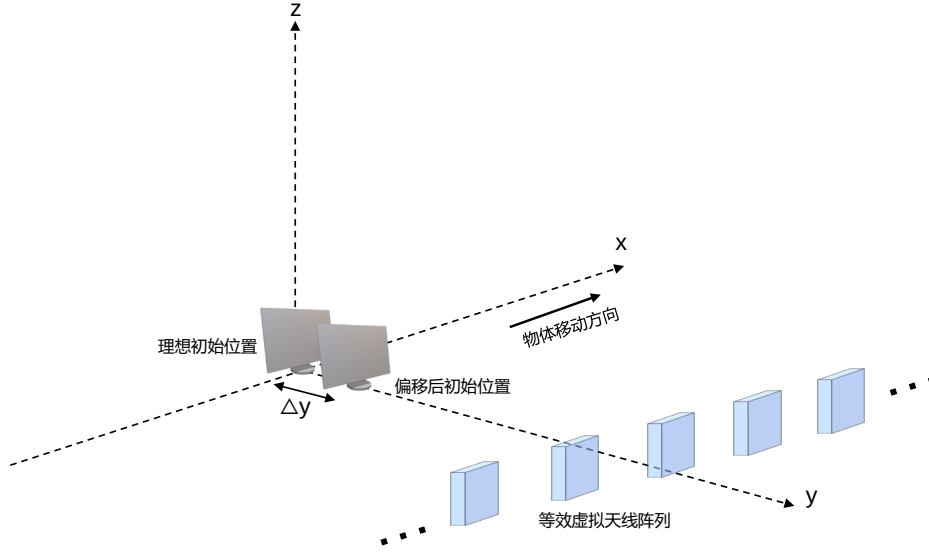
图 3-6 物体初始位置沿垂直物体运动方向发生微小位移
