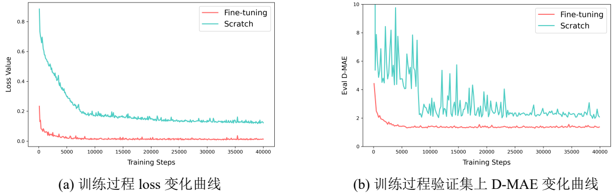
图 4-11 微调模型和从头训练的训练速度对比
