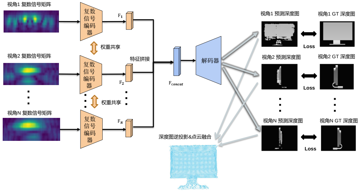
图 3-9 网络模型框架
