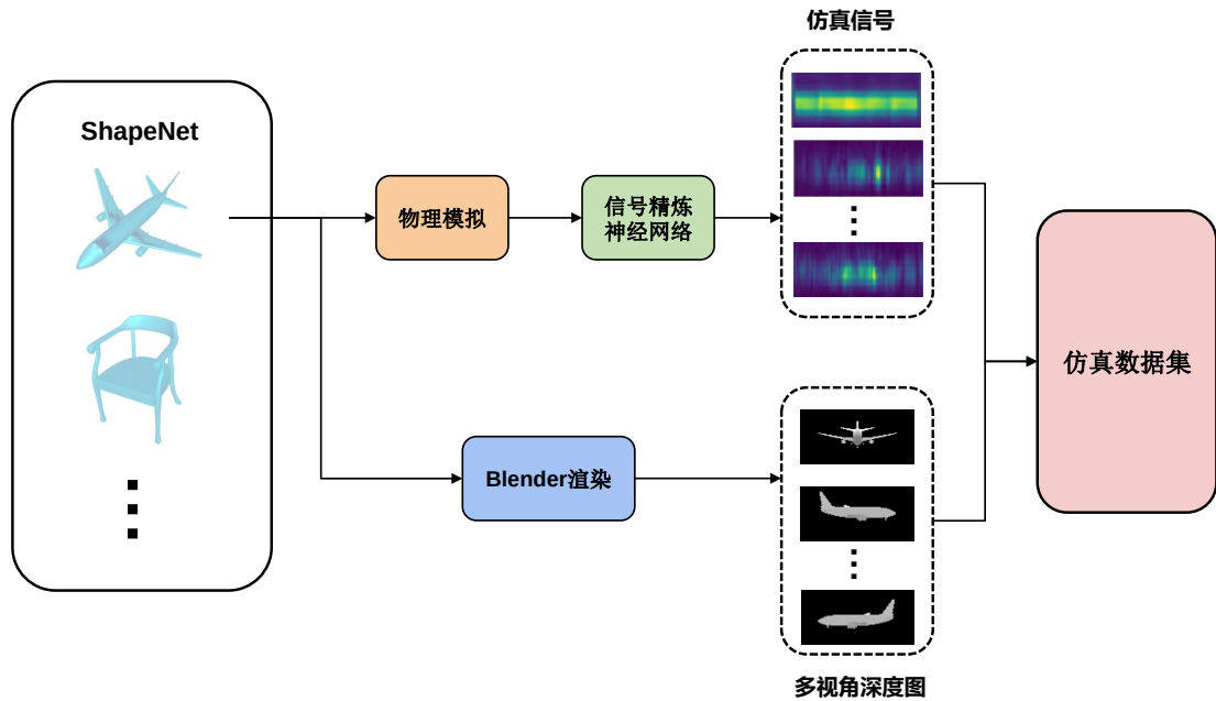
图 4-8 仿真数据集生成流程
