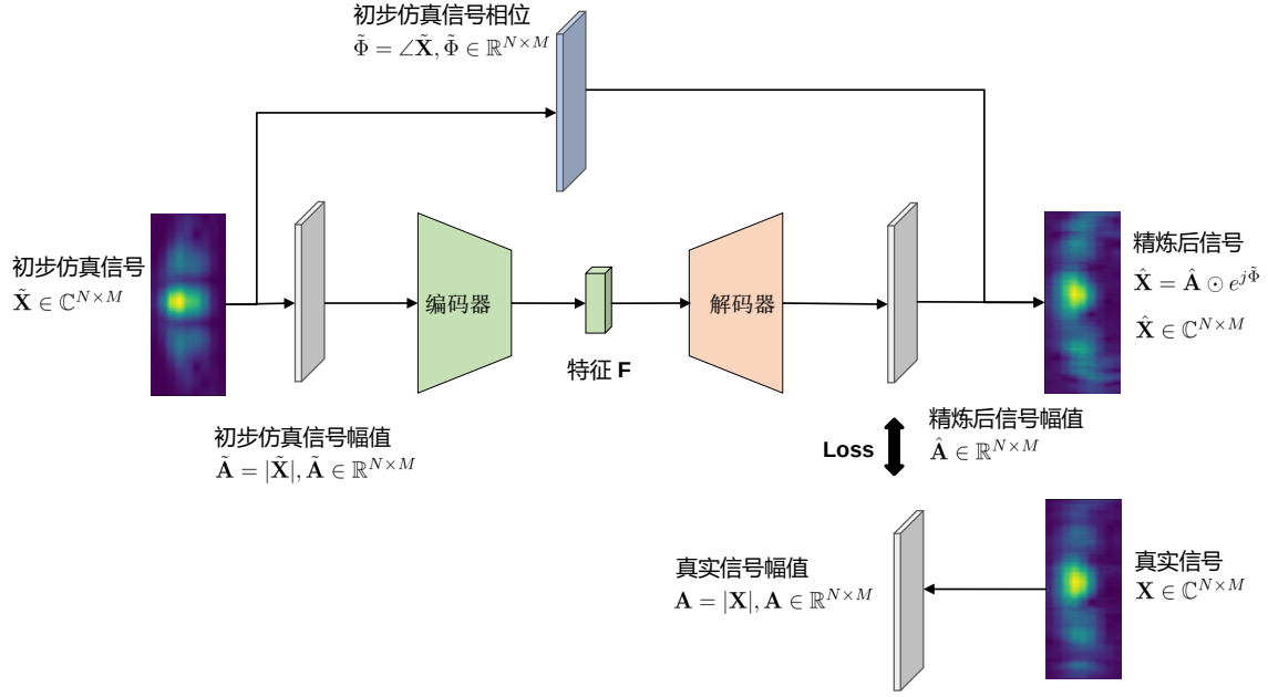
图 4-5 信号精炼神经网络
