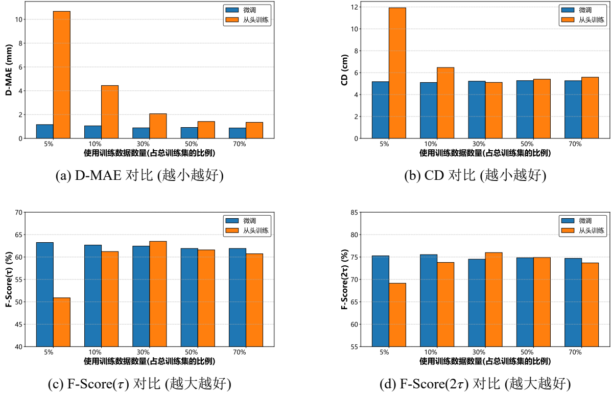
图 4-10 不同数量训练数据下微调模型和从头训练模型各评估指标对比
