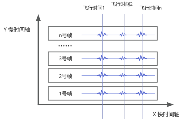
图 2-2 二维雷达信号矩阵示意图
