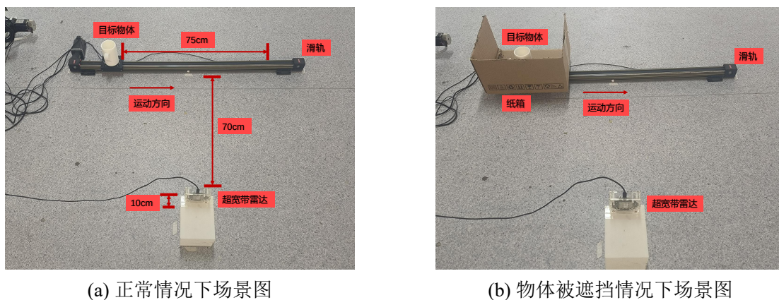
图 3-13 实验场景布置
