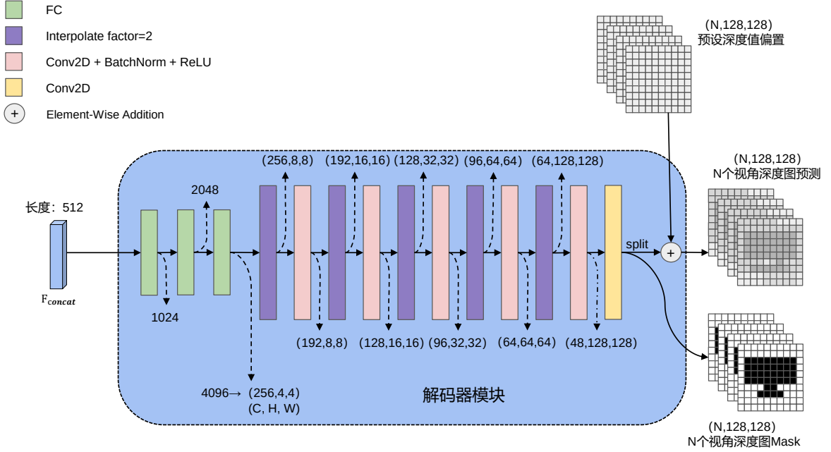
图 3-12 解码器模块
