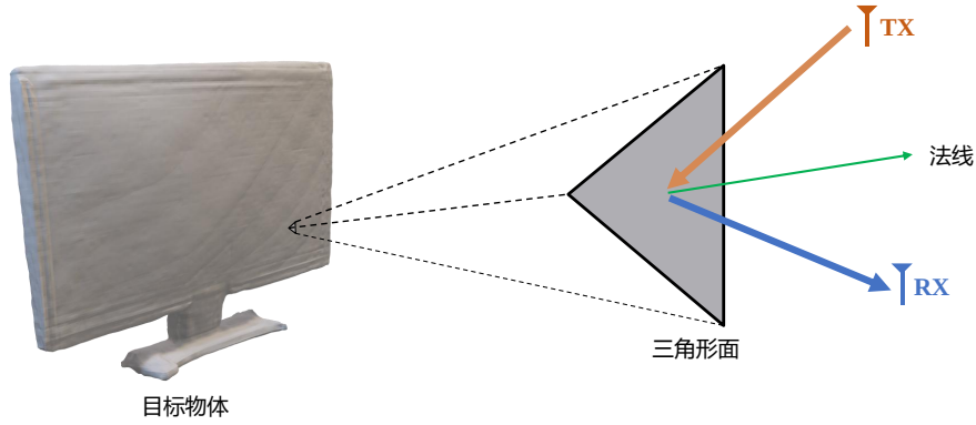
图 4-1 三维物体雷达信号模拟
