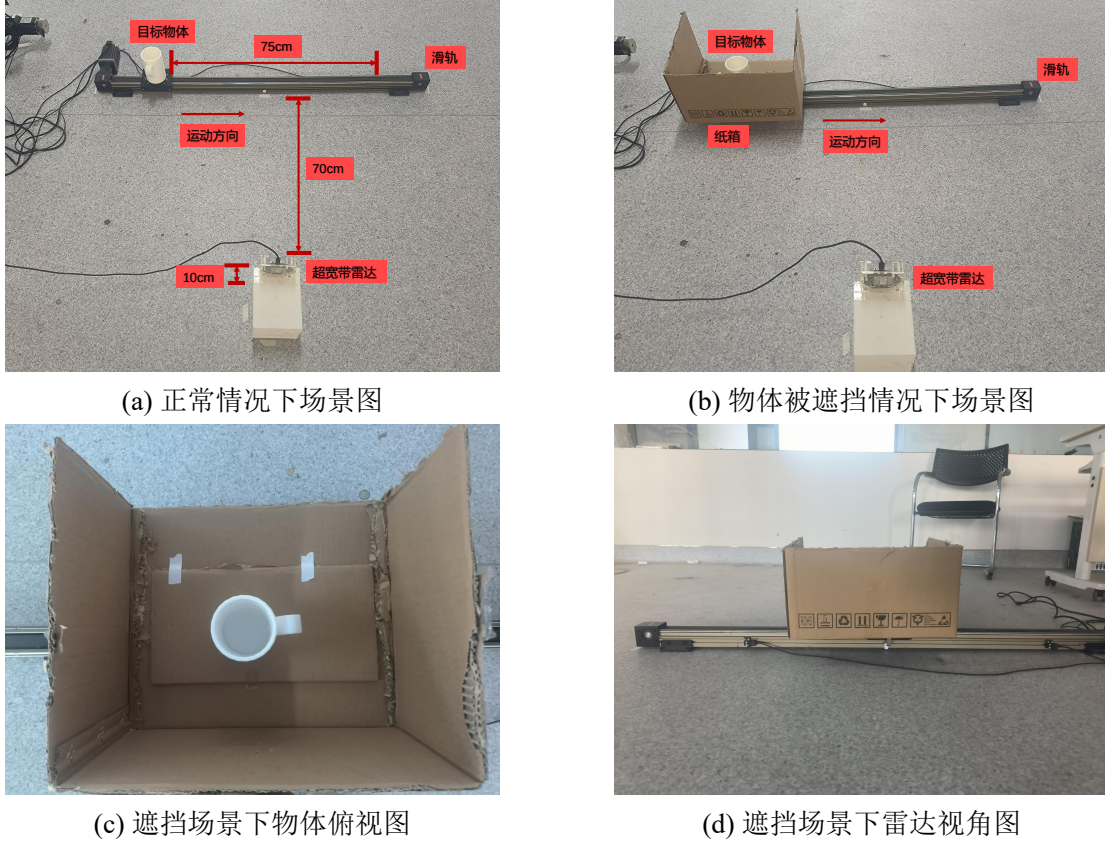
图 3-13 实验场景布置
