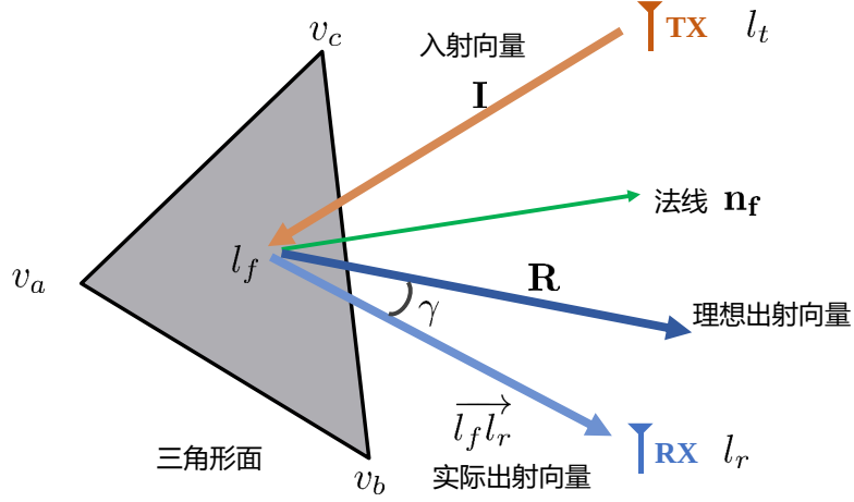
图 4-2 三角形面与收发天线的位置关系
