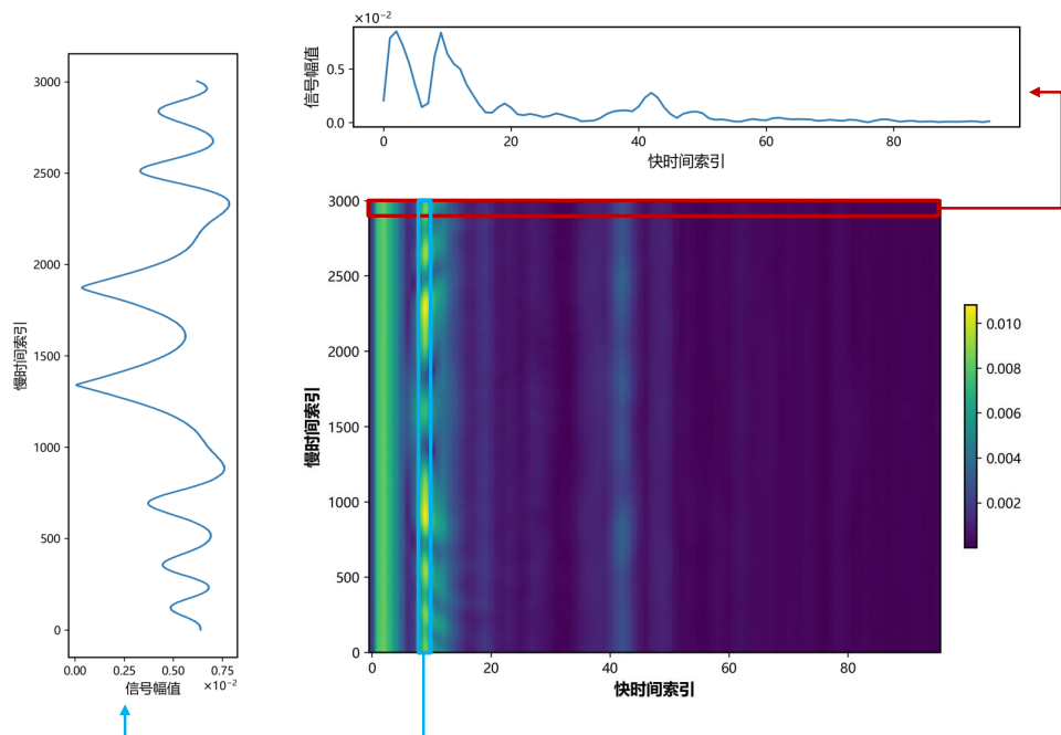
图 2-2 真实雷达信号数据幅值热图
