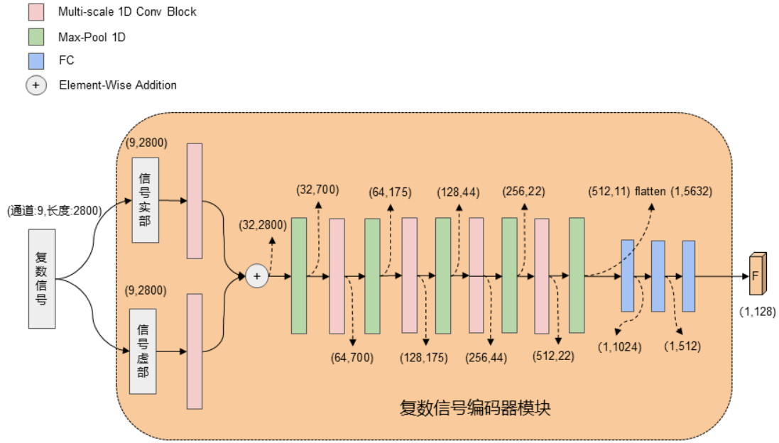
图 3-2 复数编码器模块
