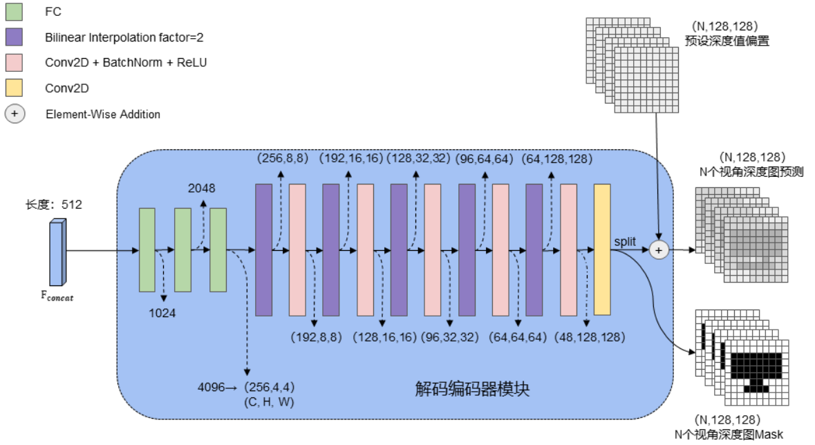
图 3-4 解码器模块
