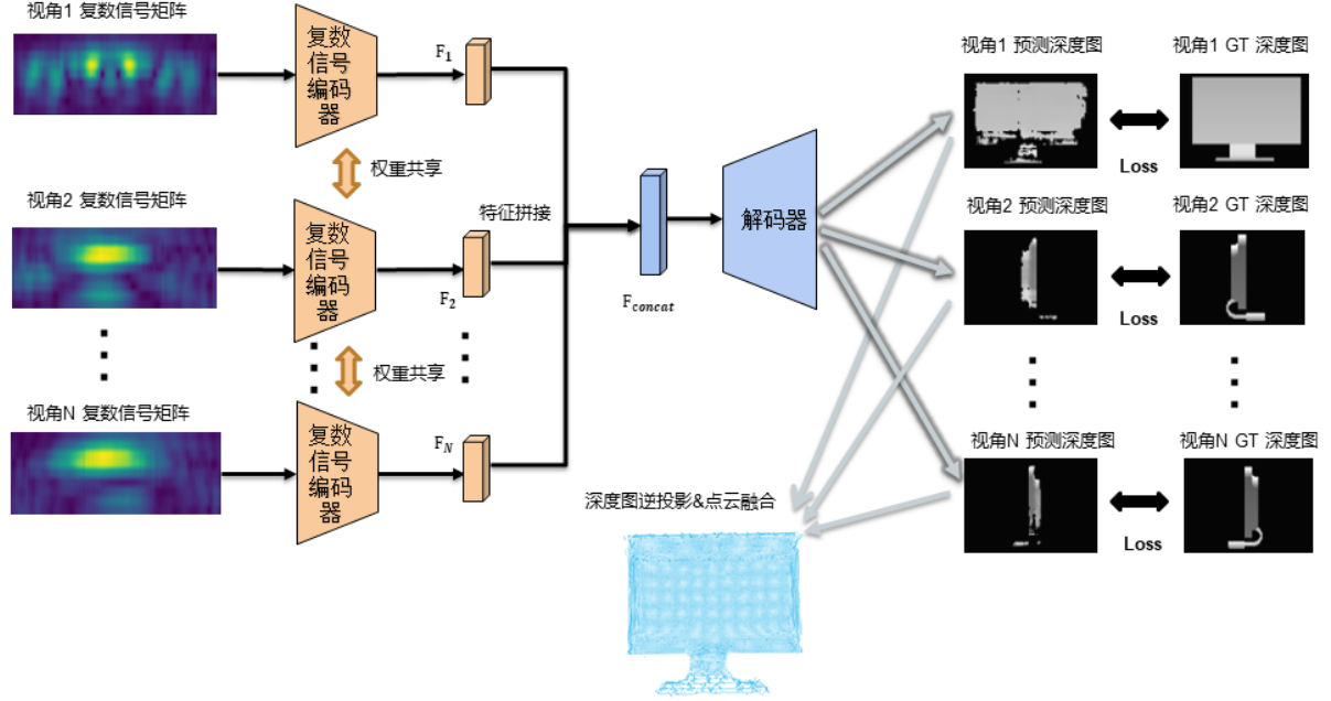
图 3-1 网络模型框架
