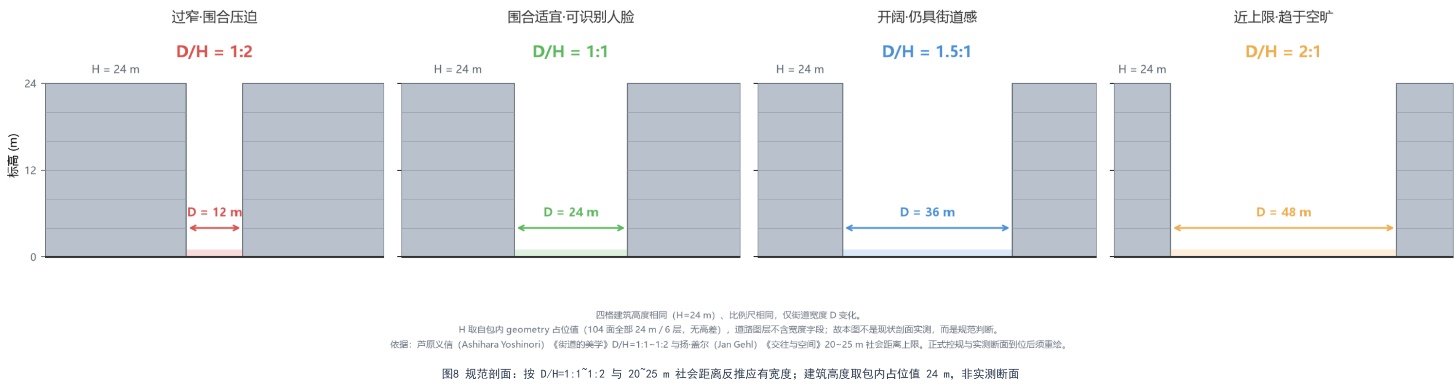
街道剖面规范研究 — 由采纳的 D/H 标准反推应有街道宽度（非实测）（v1.13）
