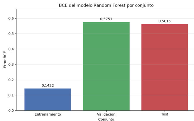
Fig. 4. Error BCE del modelo de Random Forest
