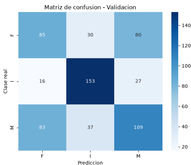
Fig. 5. Matriz de confusión del modelo Random Forest
