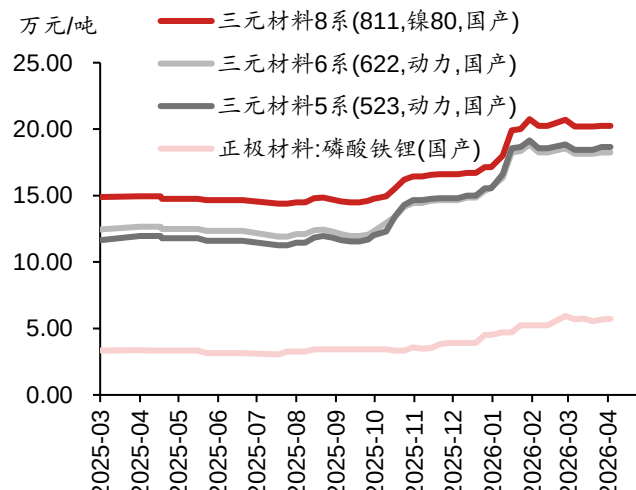
图表 9：中国三元与铁锂正极材料价格
