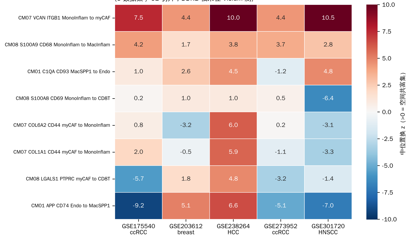
图5 Visium 跨切片空间共定位置换检验 (5 数据集 / 61 切片; DDR1 轴未在 Visium 测)
