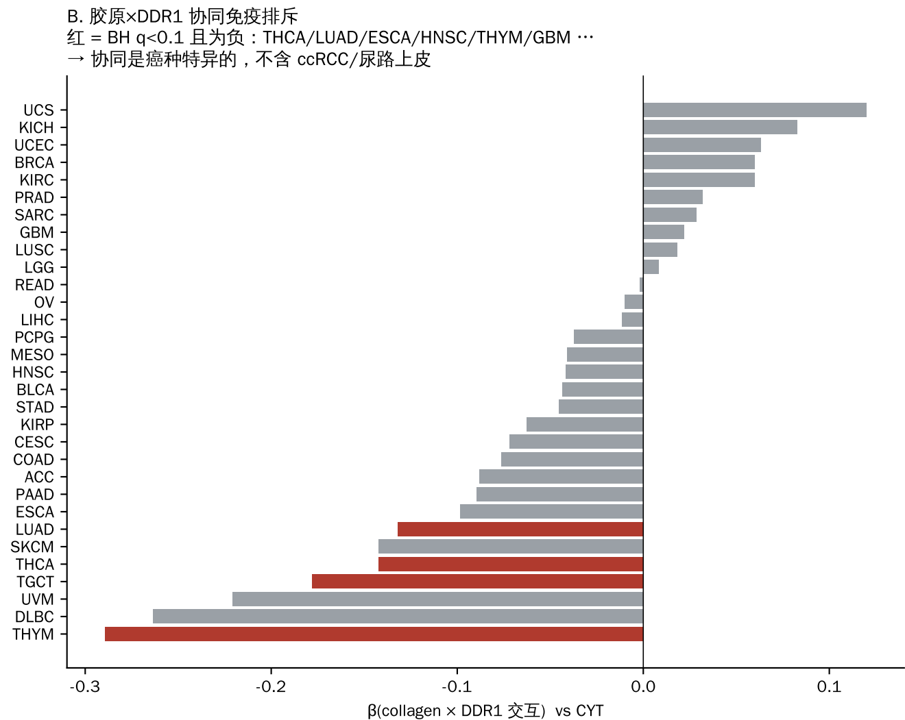
图8 TCGA 每癌种 受体端后果 CYT ~ 配体(collagen) × 受体(DDR1)
