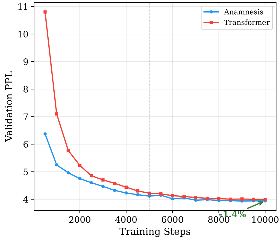
WikiText-2
