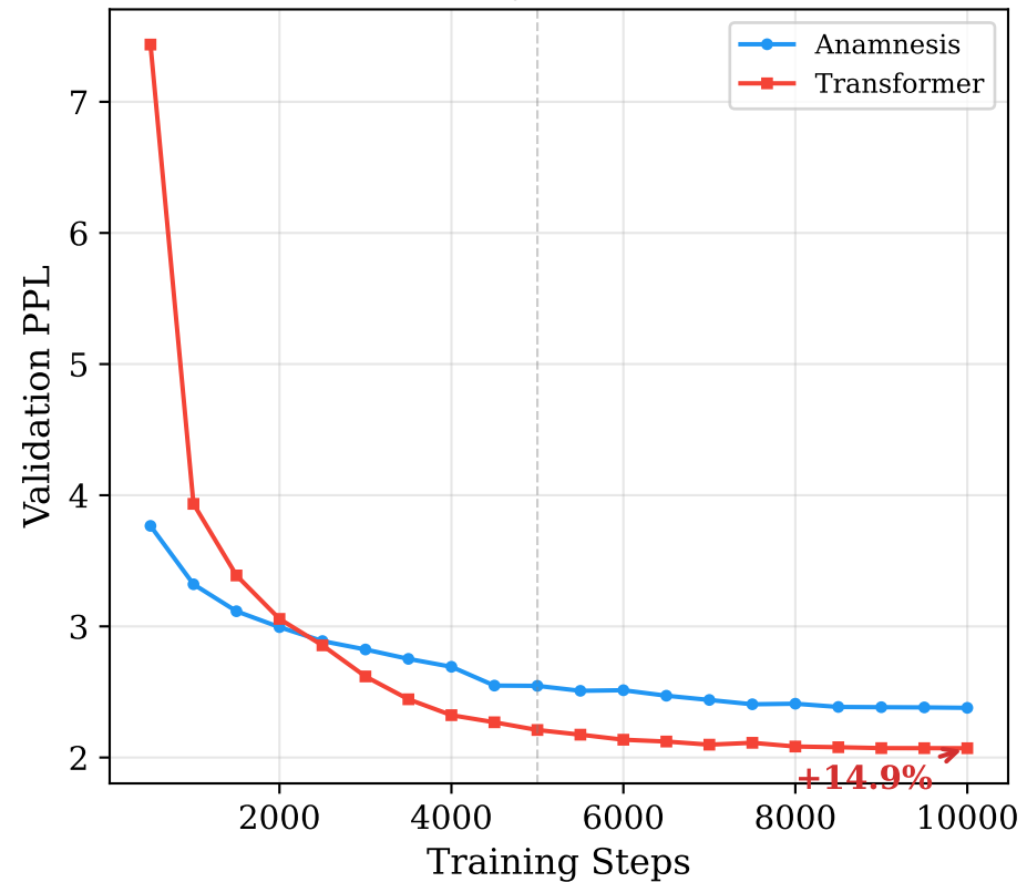
TinyStories
