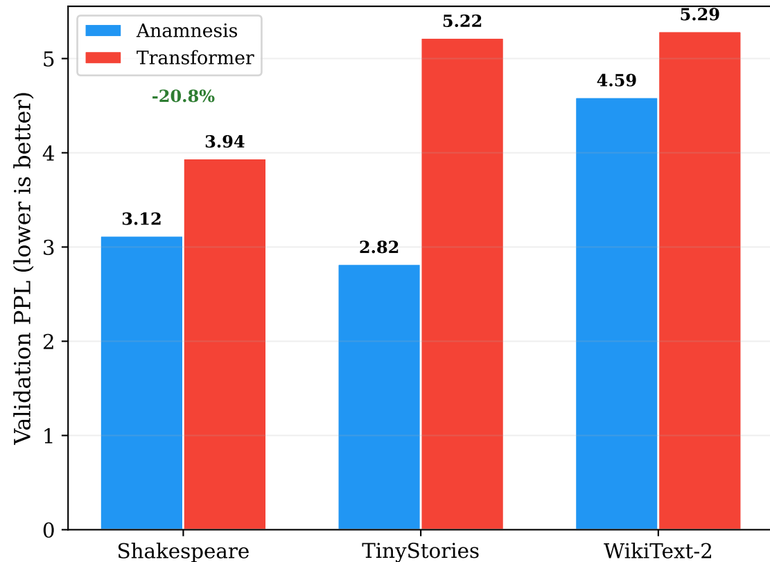
Char-level: Anamnesis vs Transformer
