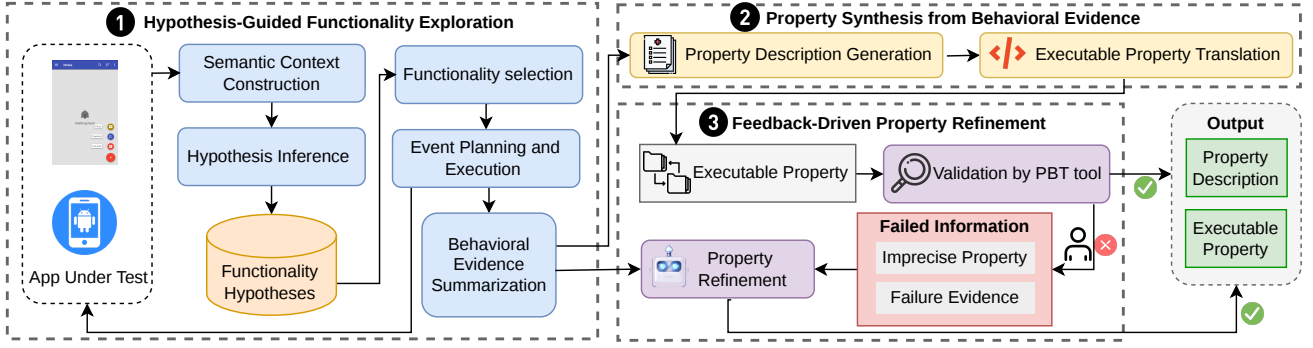
Figure 1: Overview of PROPGEN.
