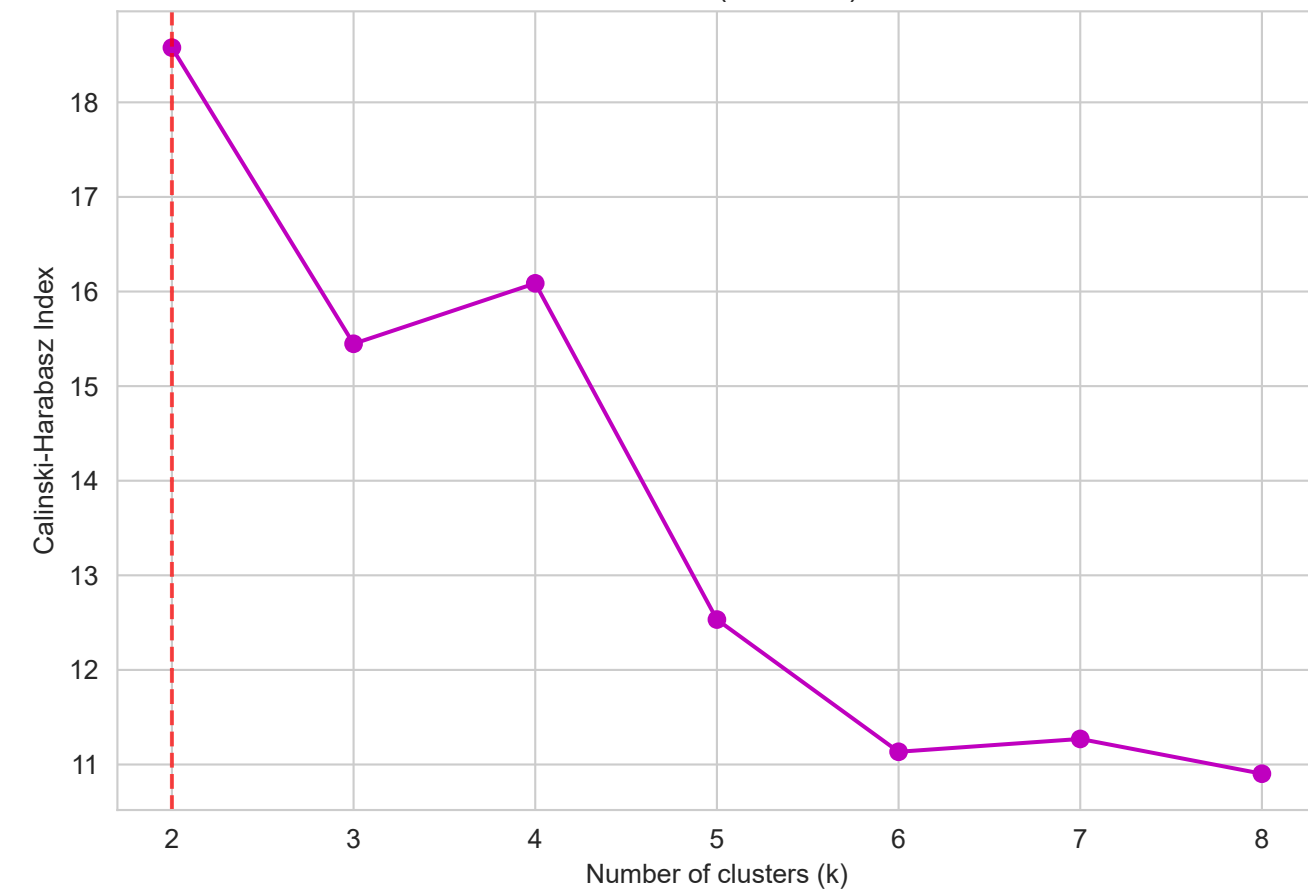
CH Index (best k=2)
