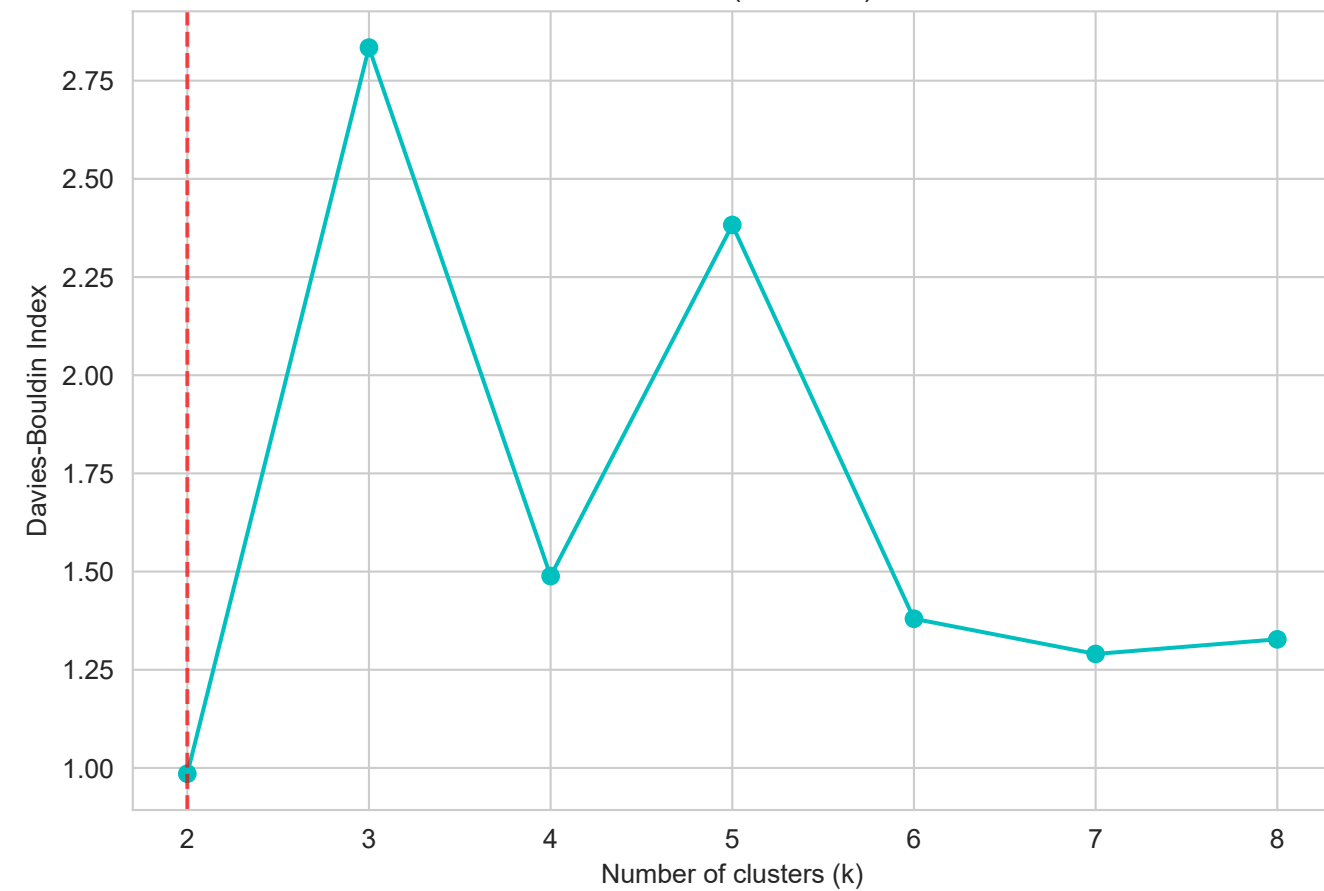
DB Index (best k=2)
