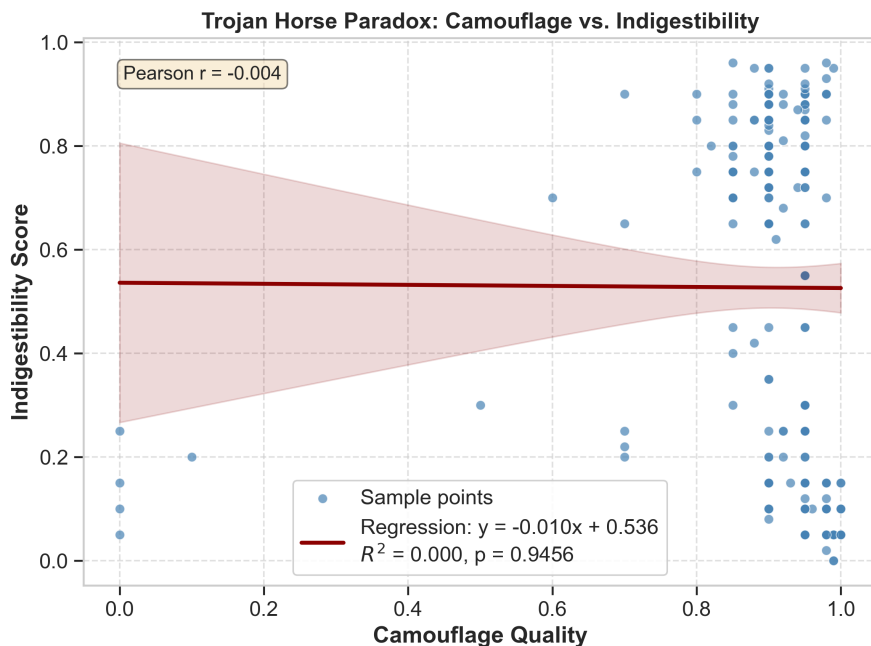
图 4-1: 伪装质量与不可消化指数的线性散点分布图
