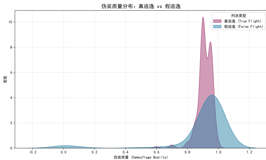
图 4-3: 真假逃逸样本的伪装质量核密度（KDE）分布与方差鸿沟
