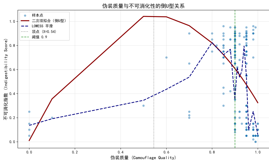
图 4-2: 伪装质量与不可消化性的倒 U 型回归曲线
