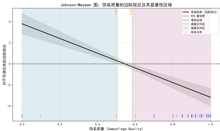
图 4-4: 伪装质量边际效应的 Johnson-Neyman 置信带分析图
