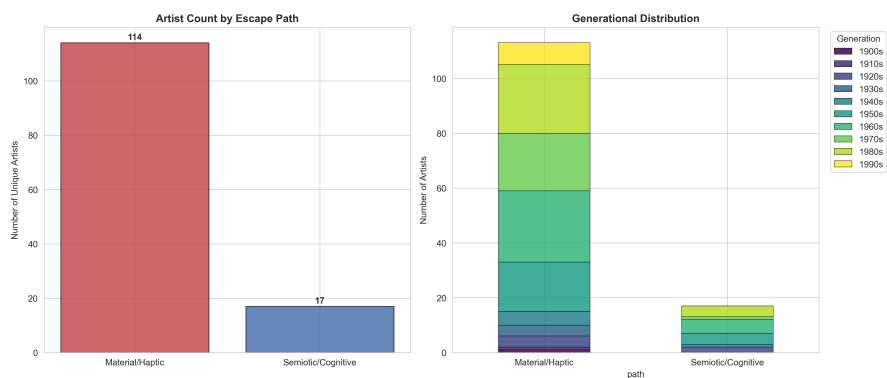
图 4-8: 两条逃逸路径中艺术家的代际与地缘拓扑对比
