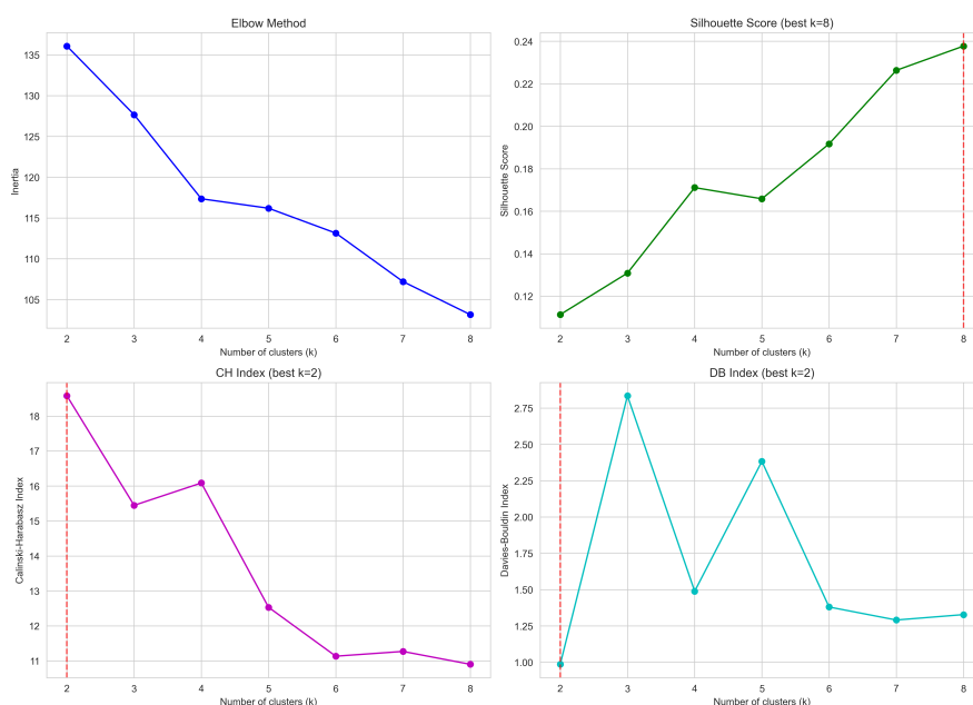
图 4-5: 聚类数验证综合指标图（肘部法则、轮廓系数、CH 指数与 DB 指数）
