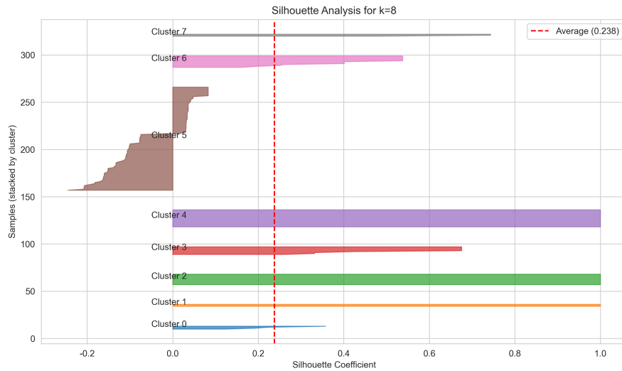
图 4-6: k=8 时的详细轮廓系数分布图 (Silhouette Distribution)
