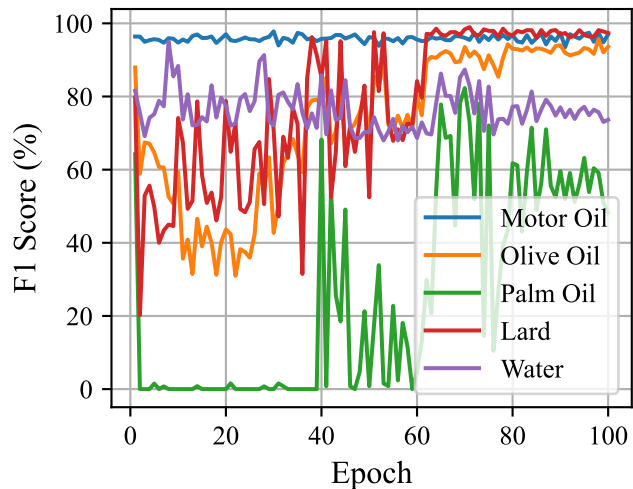
Class F1 Score
