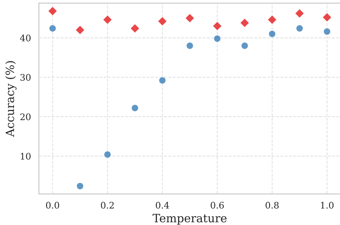
Dream-7B: MATH
