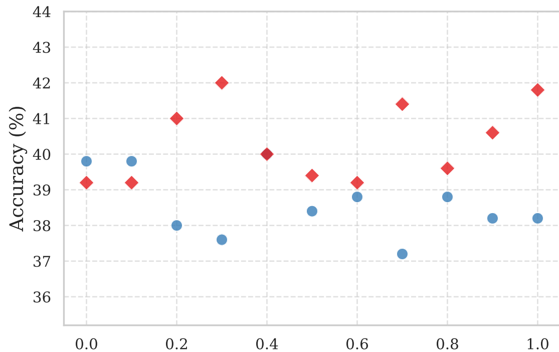
Dream-7B: MATH
