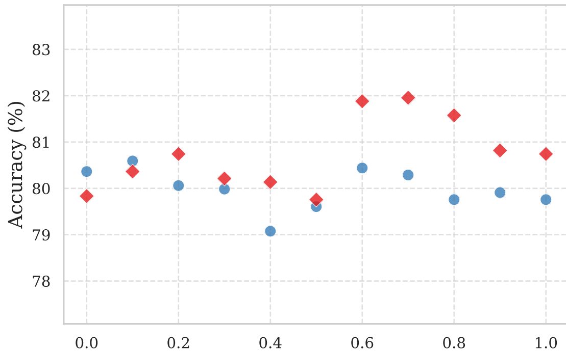
Dream-7B: GSM8K
