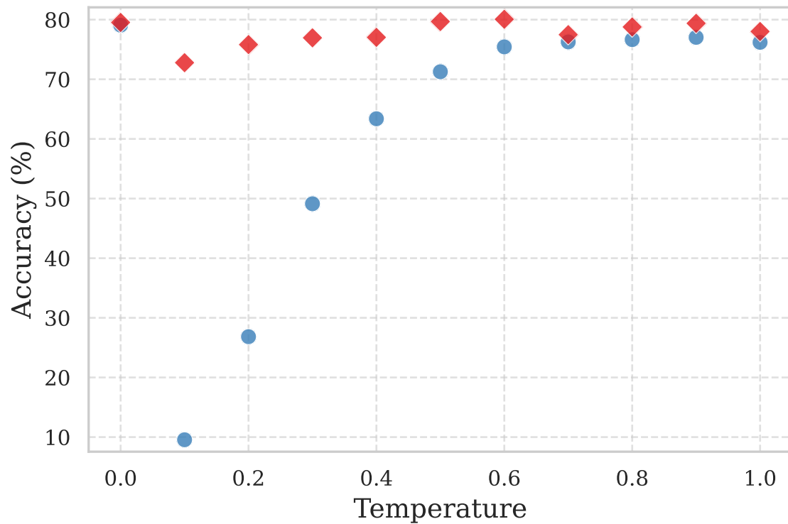
Dream-7B: GSM8K
