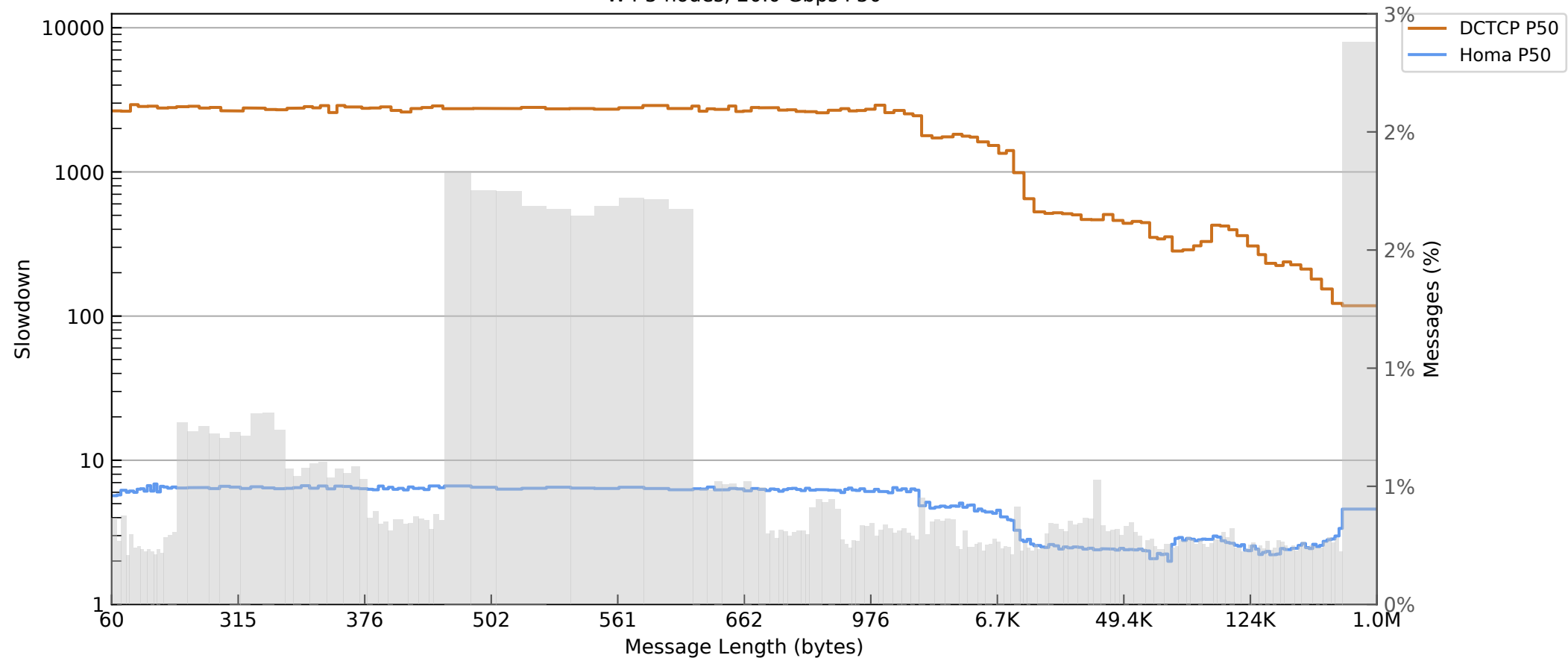
W4 5 nodes, 20.0 Gbps P50
