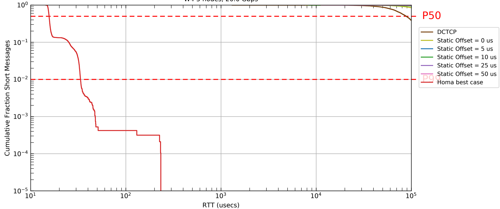
W4 5 nodes, 20.0 Gbps
