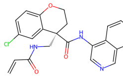
7CKT, QZU (6.06)
