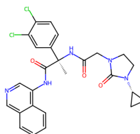
7GJU, QR5 (5.12)
