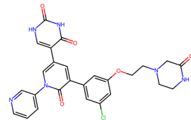
7M9Q, YTS (6.46)
