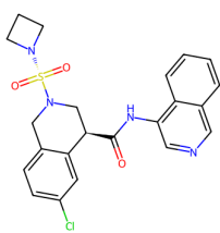
7GL3, R4X (6.8)
