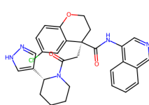
7GJT, QQU (6.28)
