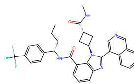
7UR4, O5O (7.45)
