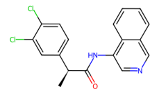
7GIQ, QH4 (6.12)
