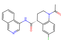
7GIZ, PUU (6.45)
