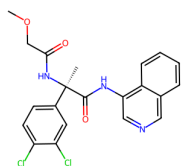
7GJR, QQF (5.03)
