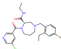
9HJH, A1IVK (6.48)
