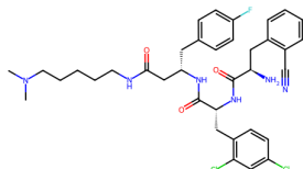
8UD0, WBK (8.0)
