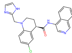
7GIP, QH7 (6.11)
