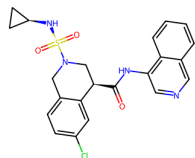
7CM5, RCX (6.95)
