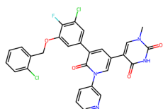
8UR9, XEK (7.36)
