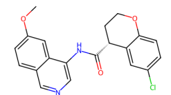
7GIW, QH6 (6.64)
