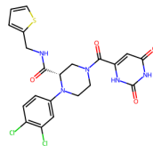
8ACD, LQ6 (6.4)
