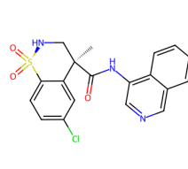
7GLW, RDK (6.58)
