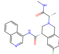
7GLZ, REU (6.91)
