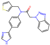
7LMF, Y6G (6.83)
