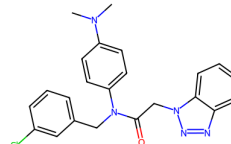
7GCF, OVF (6.3)
