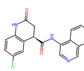
7GI8, QDF (6.35)
