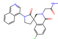
7GNC, RW9 (6.97)
