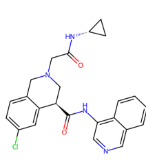
7GLE, R8O (6.92)
