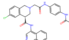
7GNQ, SSL (7.47)
