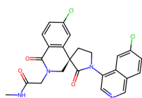
7GNI, RZF (6.84)
