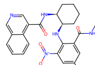
7EN8, J7R (7.14)
