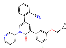
7L14, XF0 (6.77)
