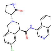
7CMO, RLR (5.91)
