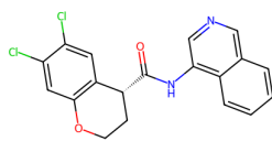
7GIO, QH4 (6.69)
