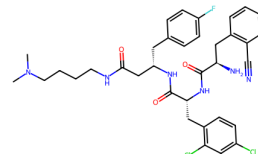
8UDP, WBO (8.0)
