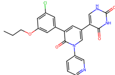
7MBM, Y5G (6.92)
