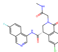
7CMW, RQ6 (6.81)
