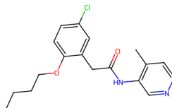
7GF5, O2R (4.61)
