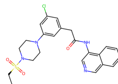
7GJJ, QO0 (5.78)
