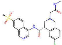
7CM6, RHl (6.71)
