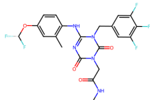
7VTH, 7XB (5.07)
