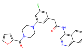
7GJZ, QRF (6.14)
