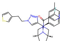
9GOI, A1IHV (6.92)
