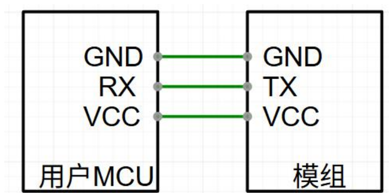
图1：系统连接图
