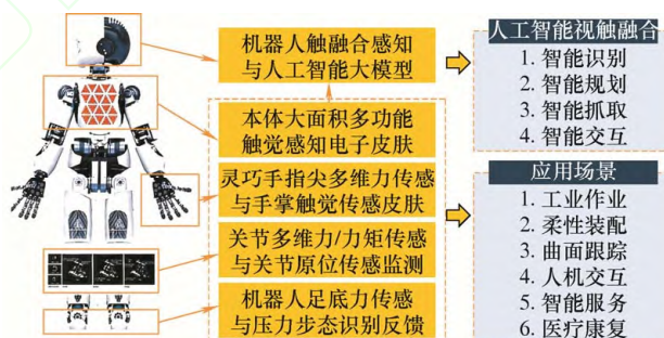
图5 人形机器人用于环境感知与场景理解的多种传感器
