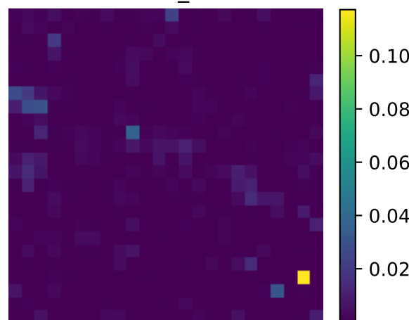
REAL P_FFN
